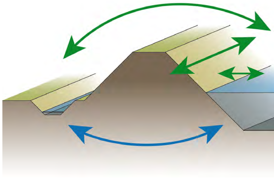
Figuur 2.1 Schematische weergave van de ecologische en hydrologische relaties van een dijk en omgeving.
