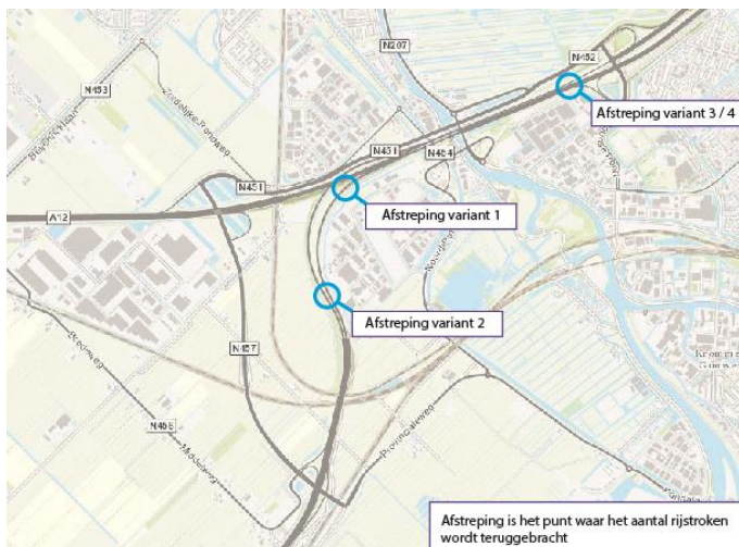
Figuur 2: Locatie van afstreping bij varianten 1 en 2 en van beëindiging derde rijstrook bij de varianten 3 en 4 schematisch weergegeven.
