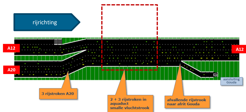
Figuur 3: Rijstrookindeling tussen de aansluiting Moordrecht (A20) en de aansluiting Gouda, richting Utrecht, op basis van variant 4 opgenomen in het voorkeursalternatief. Het rode kader geeft de positie van het aquaduct aan.
