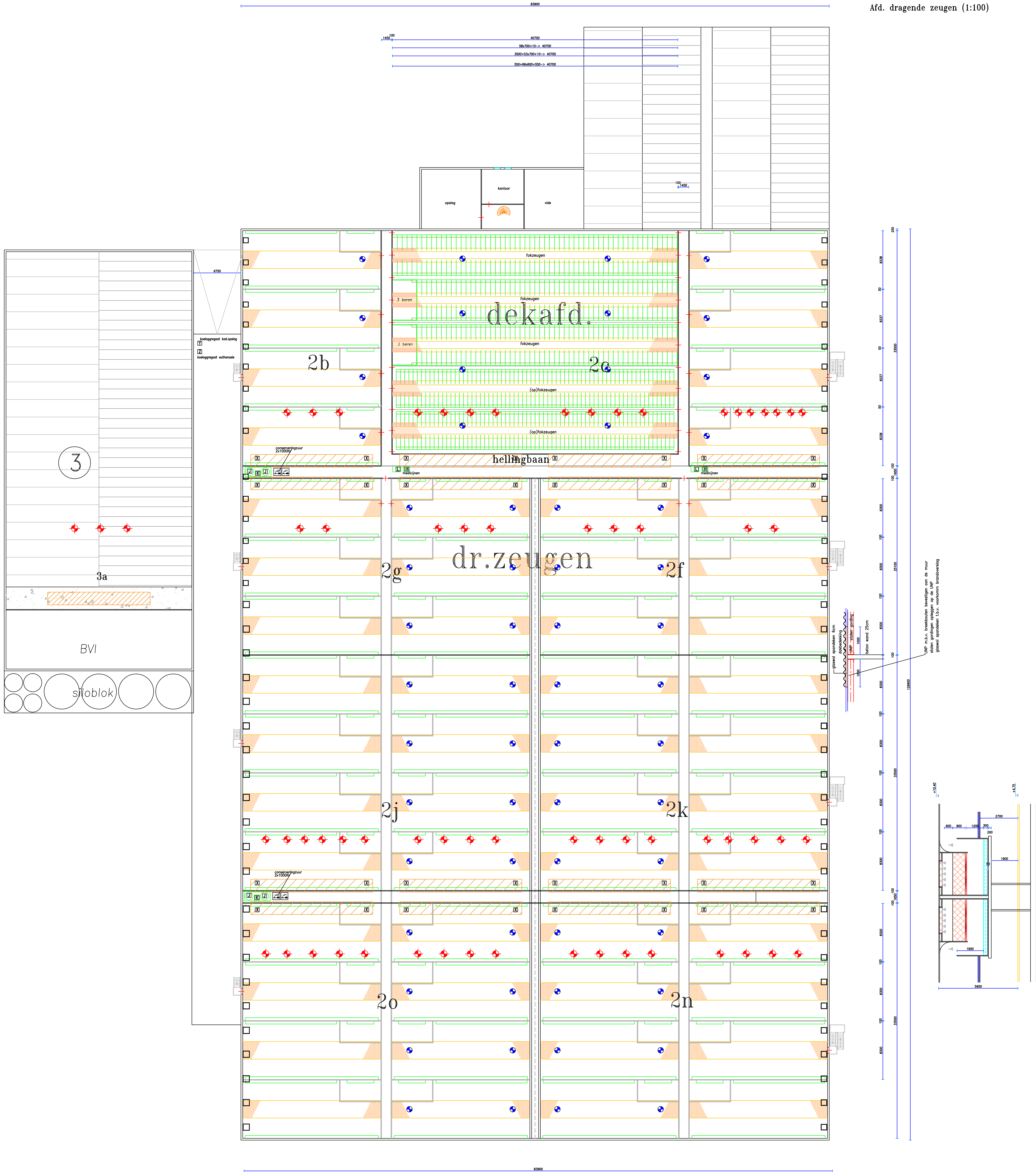
Afd. dragende zeugen (1:100)
