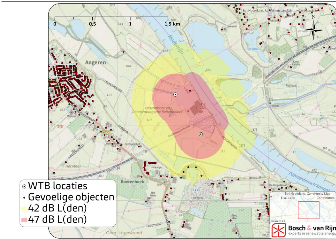
Figuur 16 Geluidscontouren variant 3
