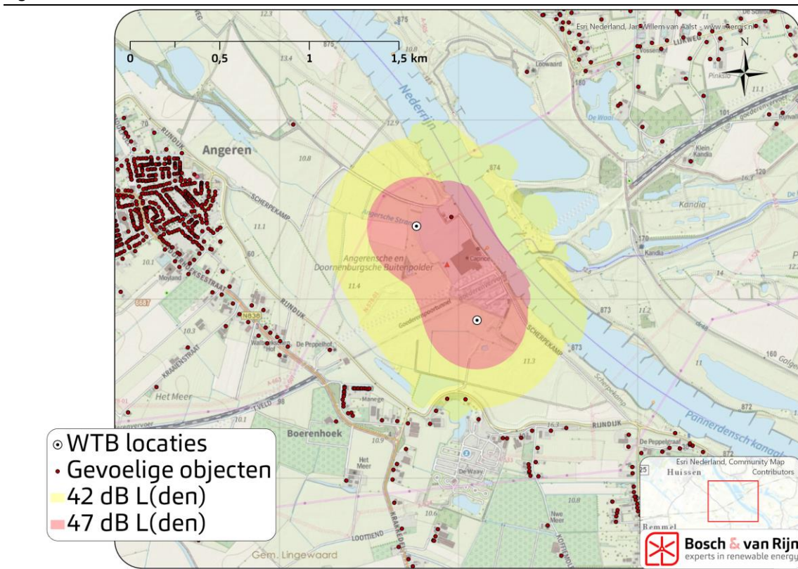
Figuur 15 Geluidscontouren variant 2
