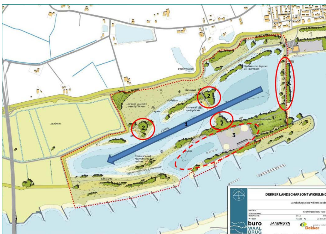
1: optimaliseren doorstromingsprofiel, 2: Oplossen van hydraulische knelpunten, 3: inpassen bedrijfsbestemming
