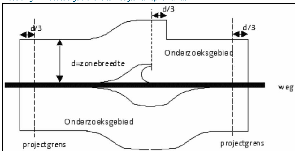
Afbeelding 2 - Illustratie geluidzone ter hoogte van op- en afritten
