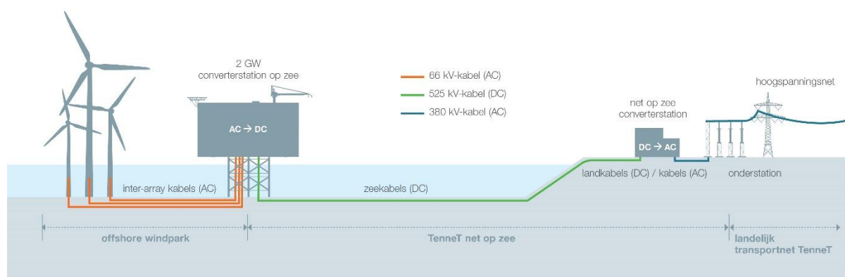
Figuur 1-2 Onderdelen project Net op Zee IJmuiden Ver Alpha
