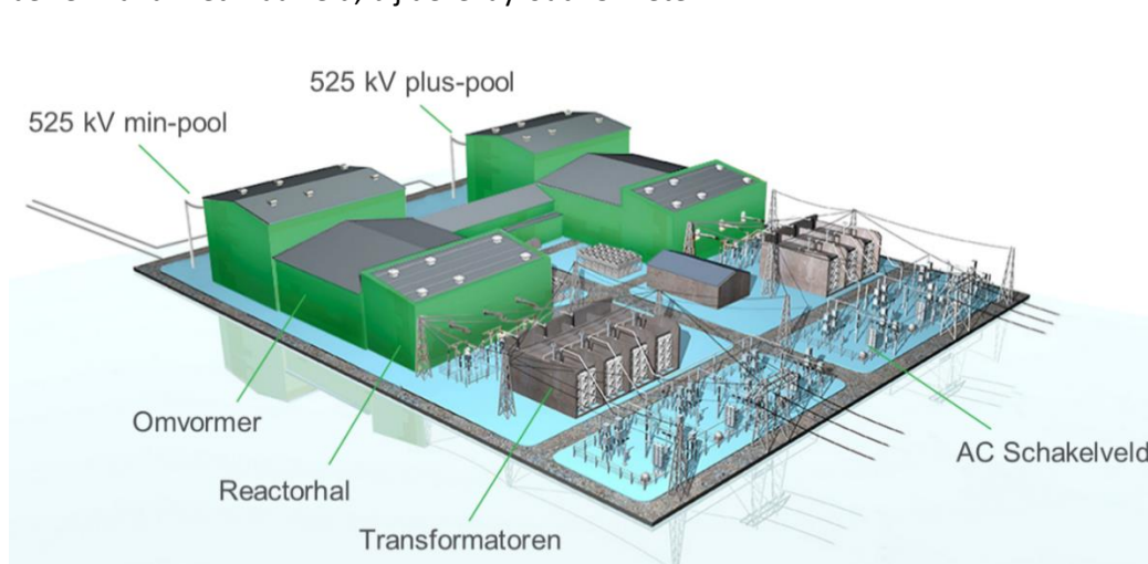
Figuur 1-9 Schematische weergave NordLink converterstation (1.400 MW)
