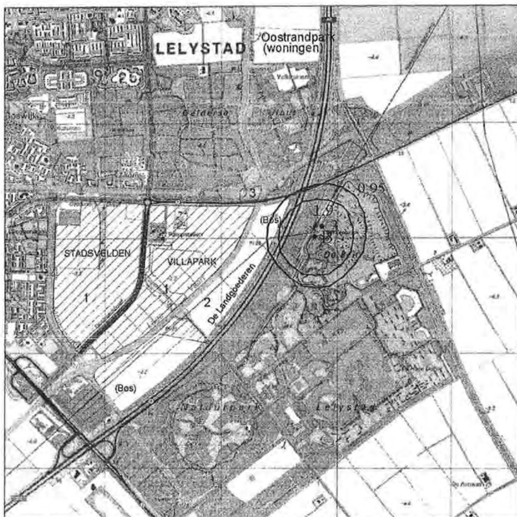
Figuur 6.1 99,5-percentiel van de uurgemiddelde geurconcentratie waarvoor geldt H=-1 ( 1,9 \text{ se}\cdot\text{m}^{-3} ) en de helft daarvan ( 0,95 \text{ se}\cdot\text{m}^{-3} ) tijdens het saneren op stortheuvel 3 en het storten in compartiment B (2010 – 2014) met het afdekken van het stortfront als reducerende maatregel. (1 rastervierkant komt overeen met 1 \text{ km}^2 )
