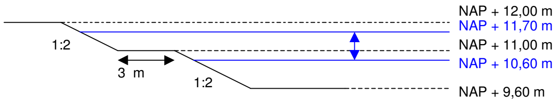
afbeelding 4.1. Profiel vijver Parallelweg
