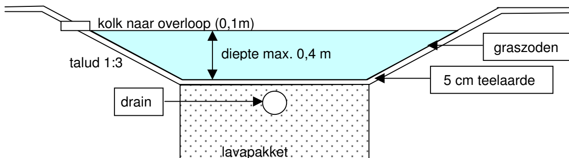
afbeelding 4.4. Dwarsprofiel wadi
