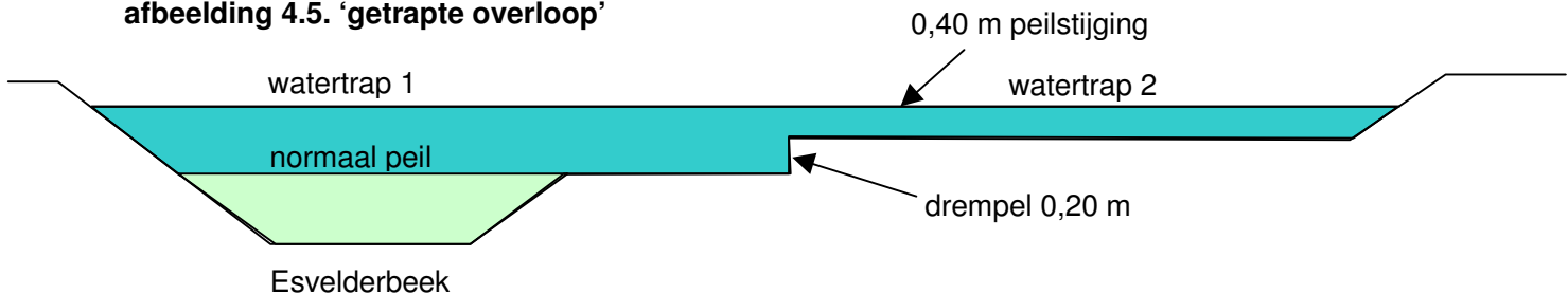
afbeelding 4.5. 'getrapte overloop'
