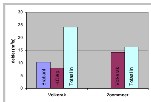
Figuur 4.2 Waterbalansen van het Krammer-Volkerak en het Zoommeer gemiddeld over de periode 1989-2000
