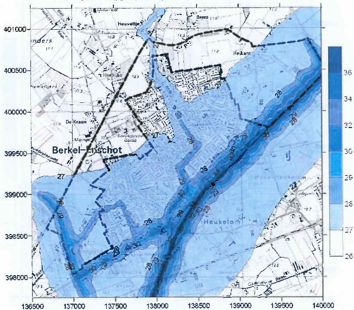
1. Contourplot NO 2 (µg/m 3 ): huidige situatie, 2004
