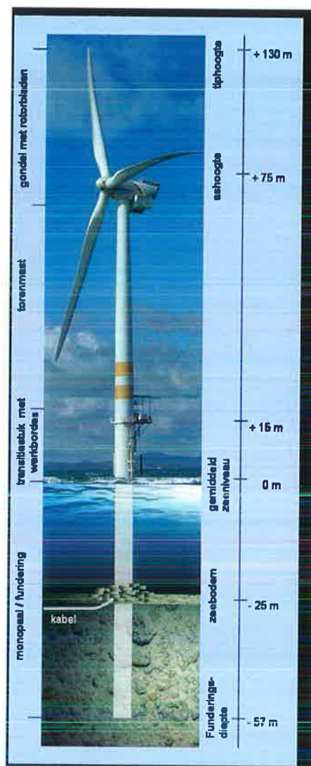
Figuur 3: opbouw van de windturbine (3.6 MW)
