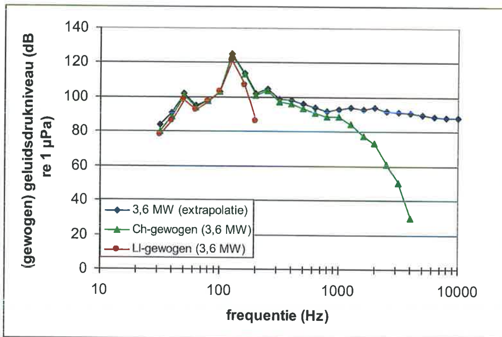
Figuur 17: op metingen in het windturbinepark Paludans Flak gebaseerde ongewogen en audiogram gewogen geluidsdrukkniveaus in tertsbanden op 100 m van de windturbine; Ch = Haring ( Clupea harengus ); LI = schar ( Limanda limanda )
