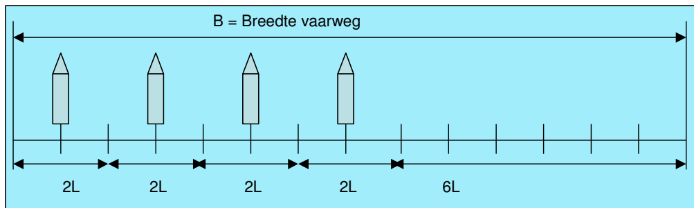
Figuur 3: De minimale breedte van een vaarweg waarin 4 schepen van 400 m lengte elkaar kunnen oplopen bedraagt 8 x de scheeps lengte ( 4 \times 2 \times 400 \text{ m.} = 3200 \text{ m.} (1,7 NM) om elkaar op voldoende afstand te passeren plus 6 scheeps lengtes voor de rondtorn (uitwijk(crash)manoeuvre) van 1 schip ( 6 \times 400 \text{ m.} = 2400 \text{ m.} (1,3 NM)) is in totaal 3,0 NM. 3
