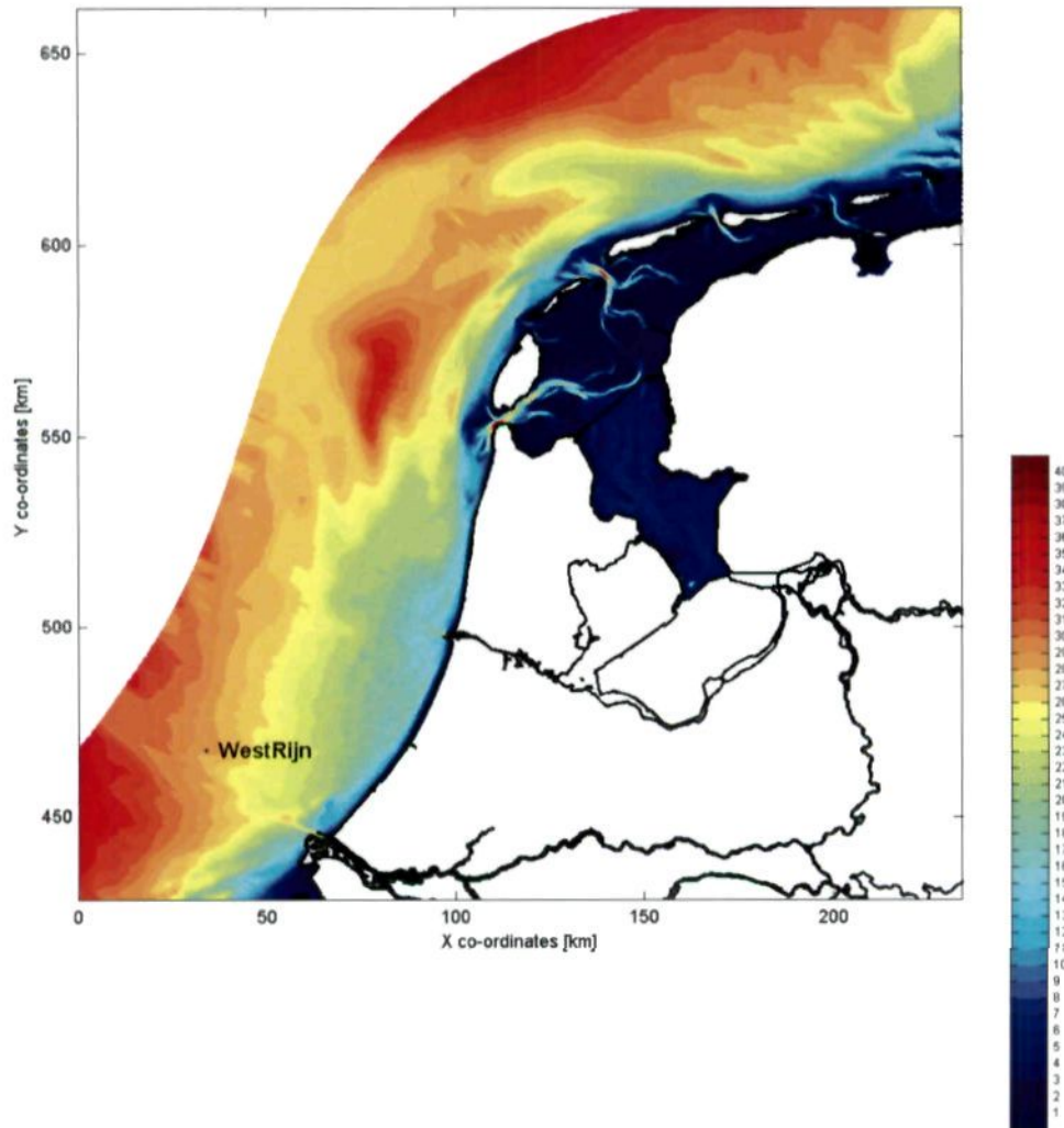
Figuur 11.1 Depth North Sea
