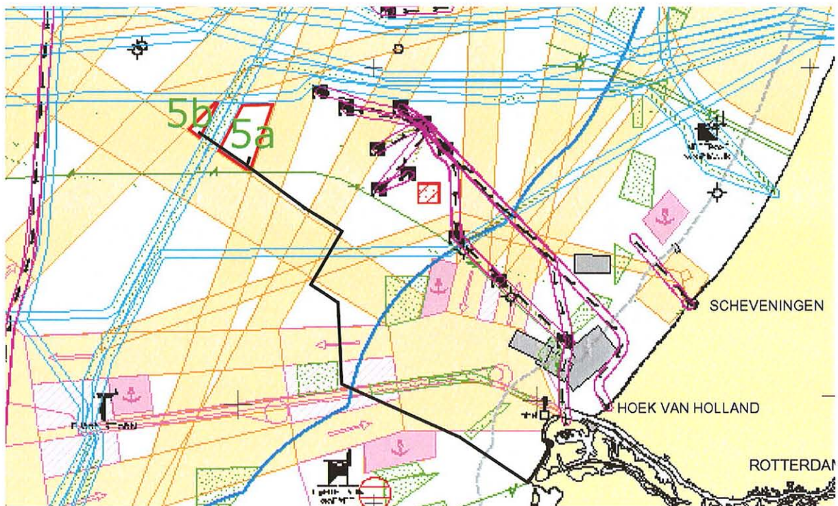
Figuur 1.1 Situering van het project Scheveningen 5 met indicatief voorkeustracé aanlandingskabel
