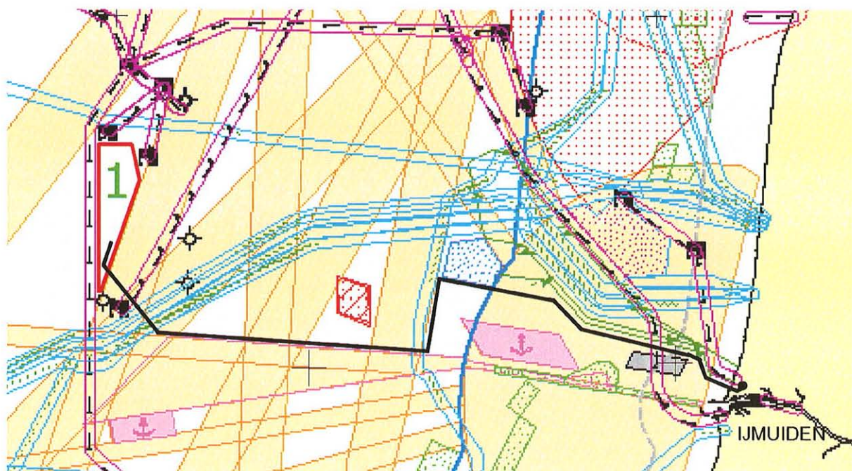
Figuur 1.1 Situering van het project IJmuiden 1 met indicatief voorkeustracé aanlandingskabel
