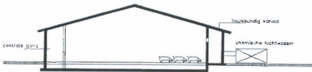
doorsnede
