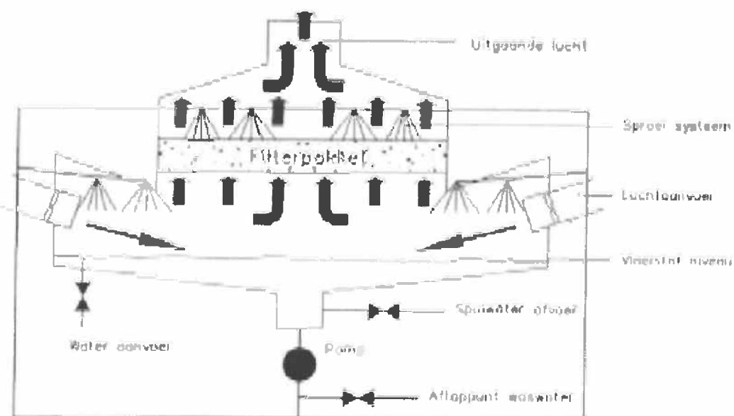
schema van biologische luchtwasser
