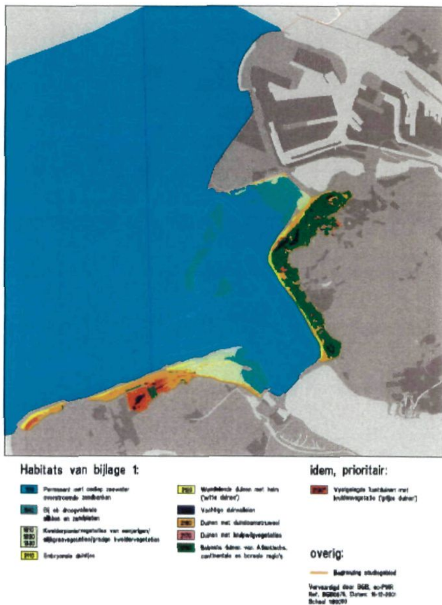
Figuur 4. Habitattypen in het kader van Natura 2000 nabij de Maasvlakte. Bron: P&R, 2001
