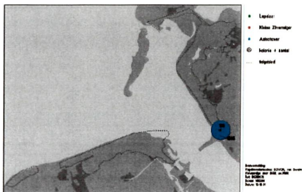
Figuur 3. Broedvogels en broedvogelaantallen in Voornes Duin. Bron: PNR, 2001
