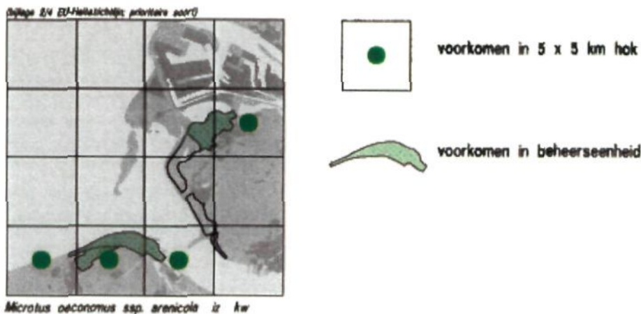
Figuur 7. Voorkomen Noordse Woelmuis: nabij de Maasvlakte. Bron: FAIR, 2001
