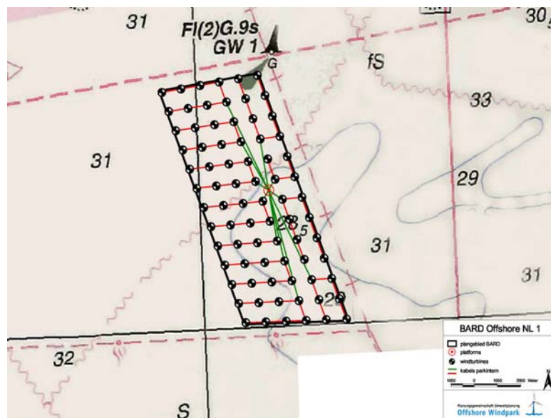
Figuur 2 Geplande opstelling windturbines, interne bekabeling en beoogde locaties voor de platforms
