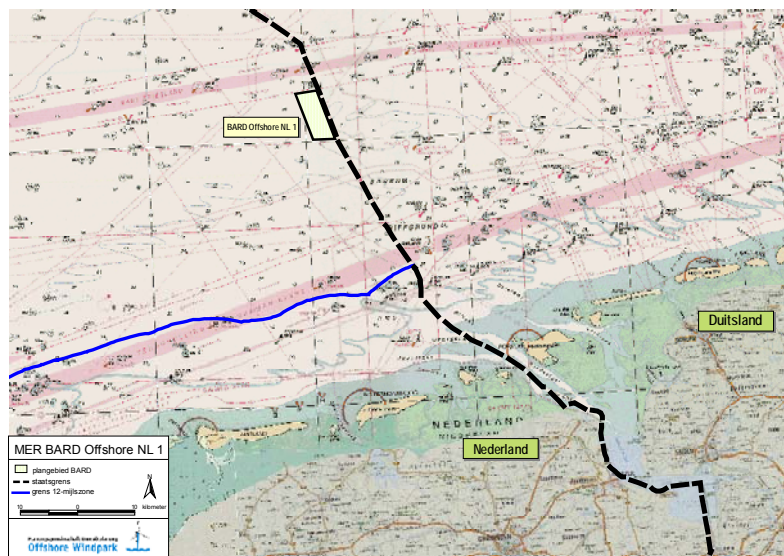
Figuur 1: Locatie van het offshore windpark BARD Offshore NL 1
