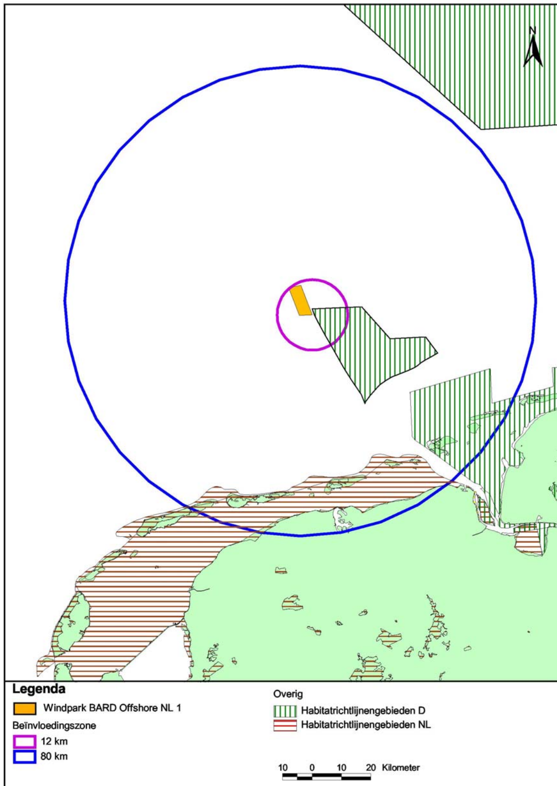
Figuur 24: beïnvloedingsgebied door heiwerkzaamheden in de aanlegfase van windpark 'BARD Offshore NL 1'
