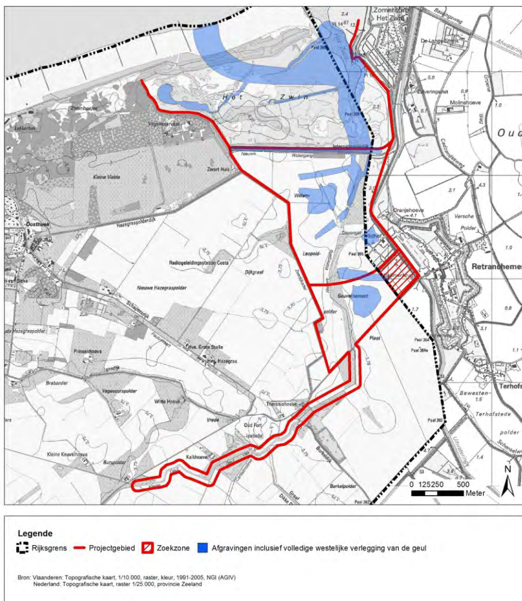
Figuur 5-5: Situering van de westwaarts verlegde Zwingseel
