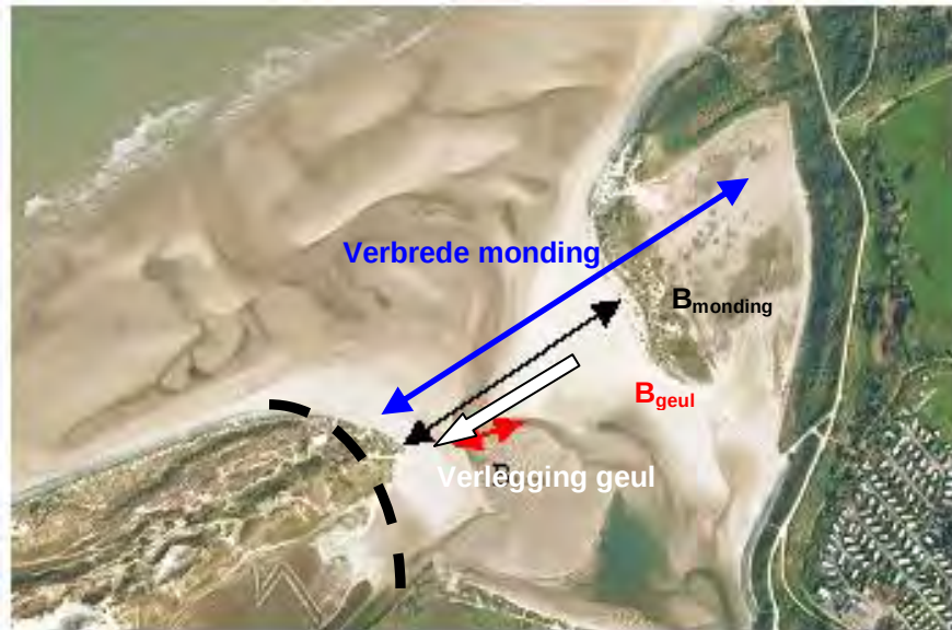
Figuur 4-4: Bovenaanzicht van de huidige toegangsgeul, met de breedte van de huidige monding tussen de duinmassieven ( B_{\text{mondig}} ), de breedte van de feitelijke toegangsgeul ( B_{\text{geul}} ), de verbrede monding en de verlegging van de geul
