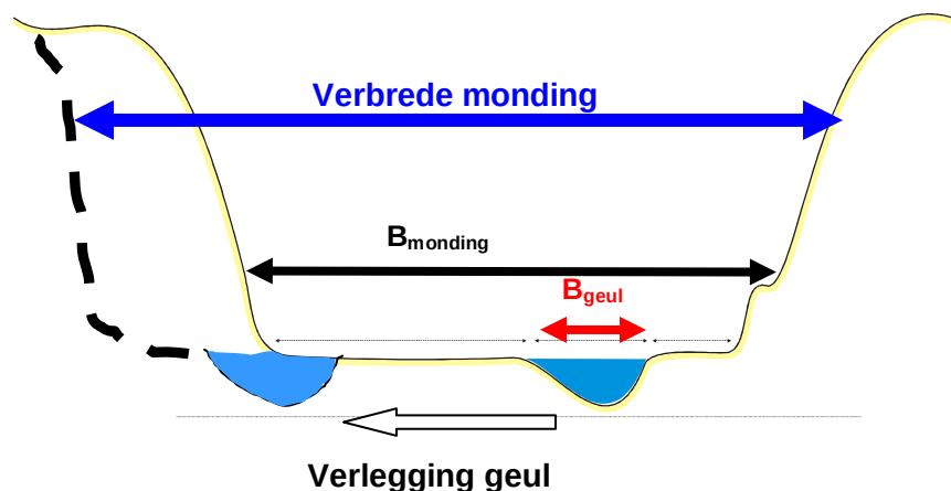
Figuur 4-5: Schematische dwarsdoorsnede van de toegangsgeul, met daarin aangegeven de breedte van de huidige monding tussen de duinmassieven ( B_{\text{mondig}} ), de breedte van de feitelijke toegangsgeul ( B_{\text{geul}} ), de verbrede monding en de geplande verlegging van de geul
