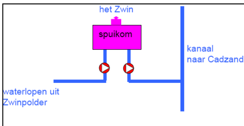
Figuur 5-15: Schematische weergave spuiwerking
