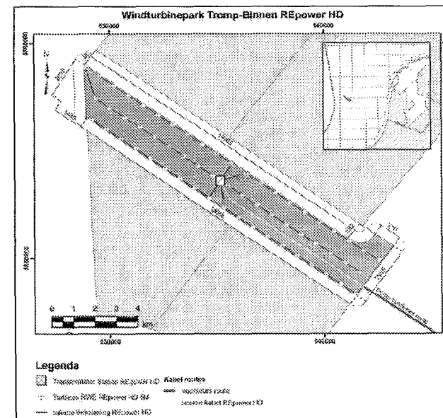
Figuur 6: Lay-out en interne bekabeling windturbinepark 'Tromp Binnen'
