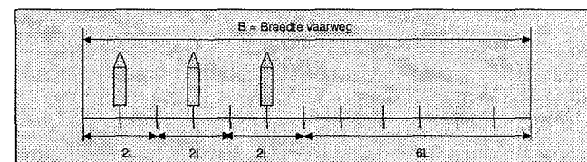
Figuur 3: Minimale breedte van een vaarweg waarin 3 schepen van 400m lengte elkaar kunnen oplopen bedraagt (3 \times 2^{10} \times 400 \text{ m}) = 2400 \text{ m} (=1,3 NM) voor het op voldoende afstand passeren van elkaar plus 6 scheepslengtes (= 6 \times 400 \text{ m} = 2400 \text{ m} = 1,3 \text{ NM}) voor de effectieve draaicirkel in geval van een uitwijk(crash) manoeuvre van 1 schip dus in totaal 2,6 NM).
