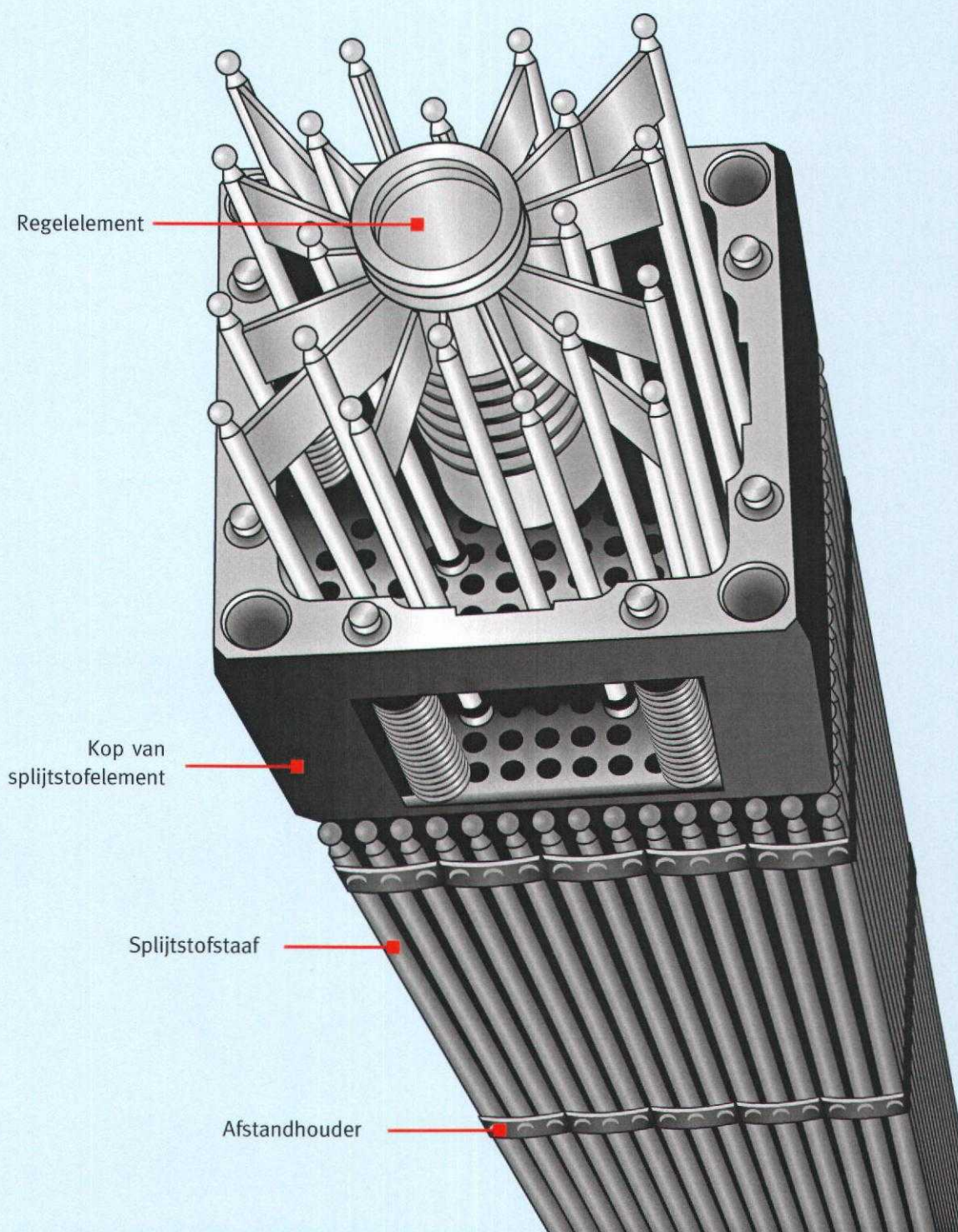
Figuur 4.3 Bovenzijde van een splijststofelement met daarin een regelement (met daarin twintig regelstaven) van de Kerncentrale Borssele
