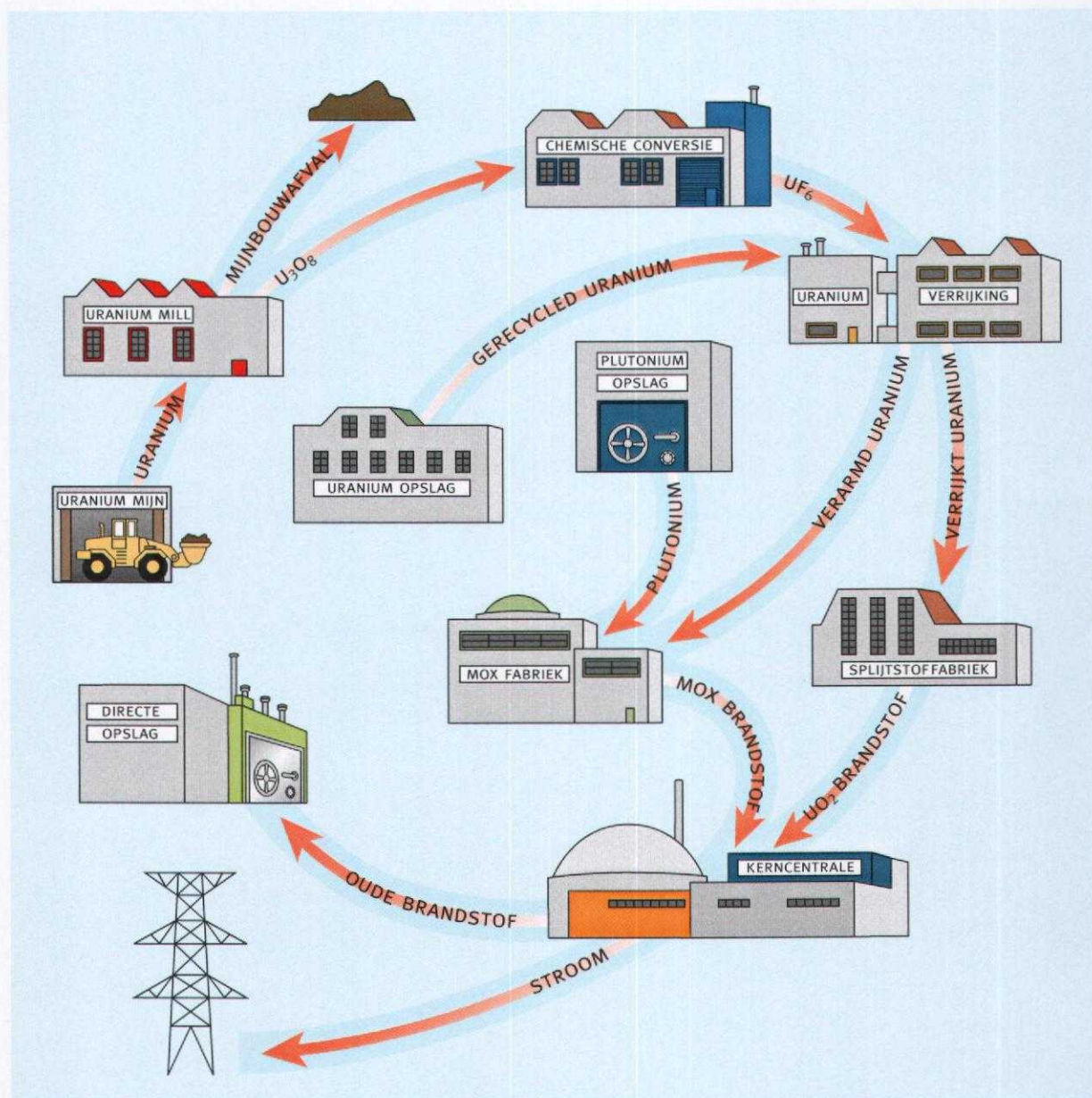
Figuur 4.5 Principeschema open splijtstofcyclus
