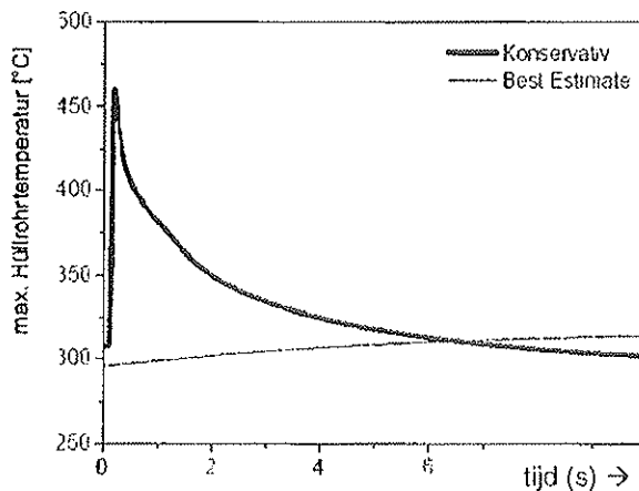
Fig. 7.5 maximale temperatuur splijstofomhulling (MOX)
