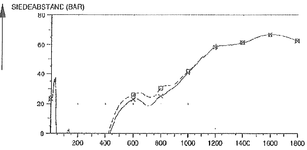
Fig. 7.13 Temperatuur primaire koelmiddel (°C) en kookafstand (bar) gedurende ATWS. Tijd is in seconden,
