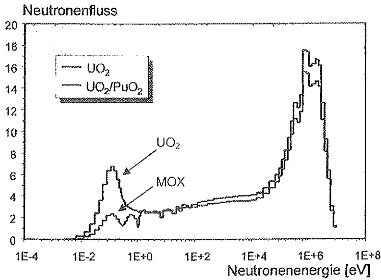
Fig. 4.5 Typische neutronenflux van een MOX splijstofelement en een UO_2 splijstofelement
