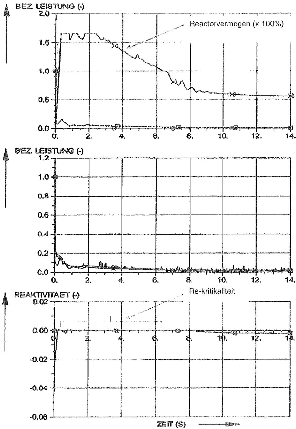
Fig. 7.1 Re-kritikaliteit MOX kern bij breuk hoofdstroomleiding t.g.v. aardbeving
