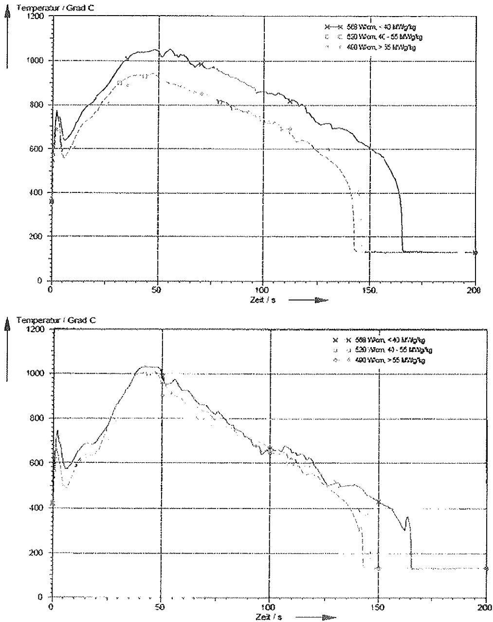
Fig. 7.9 Verloop van de temperatuur van de splijtstofomhulling (cladding) bij een groot Koelmiddel Verlies Ongeval; boven zonder opzwellen en barsten van de cladding en onder met opzwellen en barsten van de cladding
