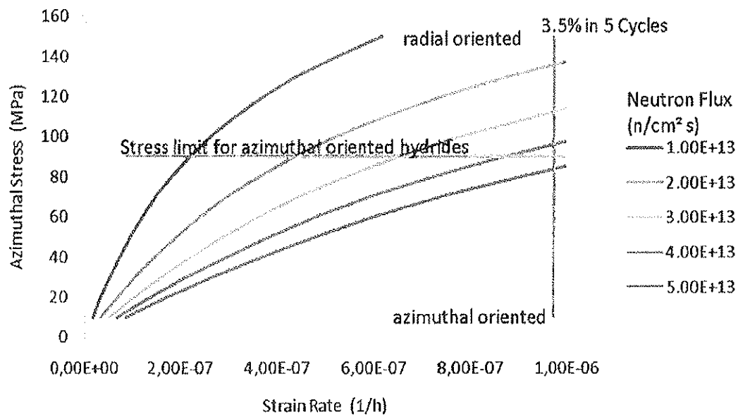
Fig. 9.1 Relatie tussen tangentiële spanning en reksnelheid als functie van de neutronenflux.
