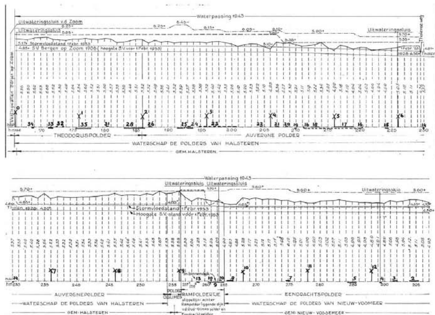
Figuur 14 Langsdoorsnede dijklichaam nabij Vossemeer (situatie 1943)
