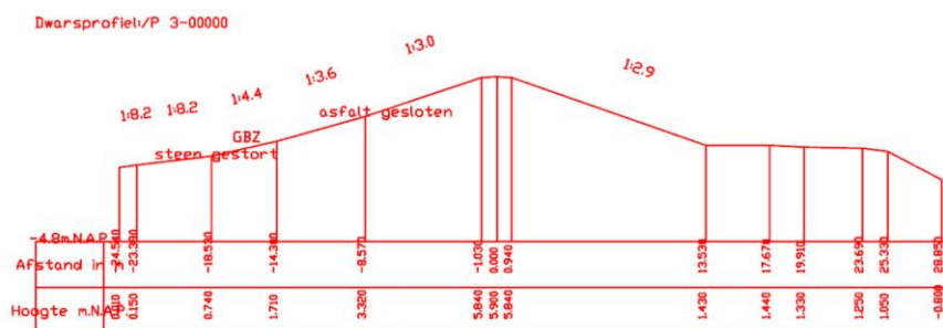
Figuur 9 Actuele hoogte, NAP + 5.9 m, hoogte 1943, NAP + 5.28 (km #10)
