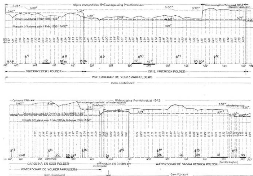
Figuur 2 Lengteprofielen Brabantse dijken in 1943
