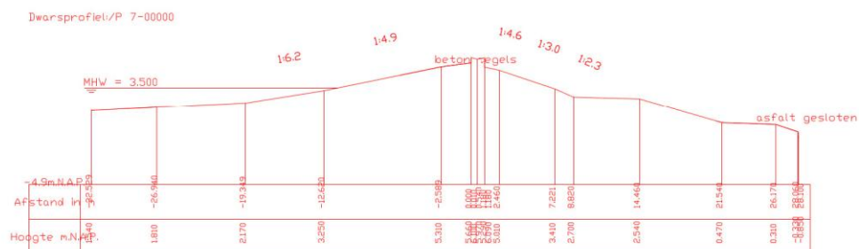
Figuur 8 Huidig dwarsprofiel ter hoogte van km 15
