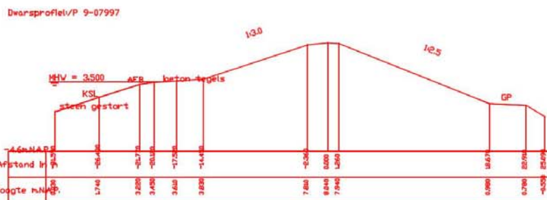
Figuur 3 Huidig dwarsprofiel ter hoogte van km 7.0
