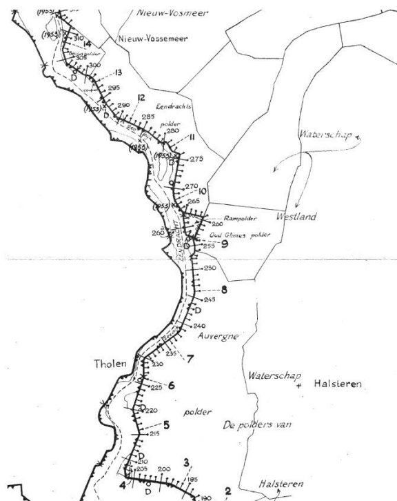
Figuur 13 Overzicht dijkkring 44 (Vossemeer)
