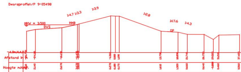
Figuur 4 Huidig dwarsprofiel ter hoogte van km 8.3
