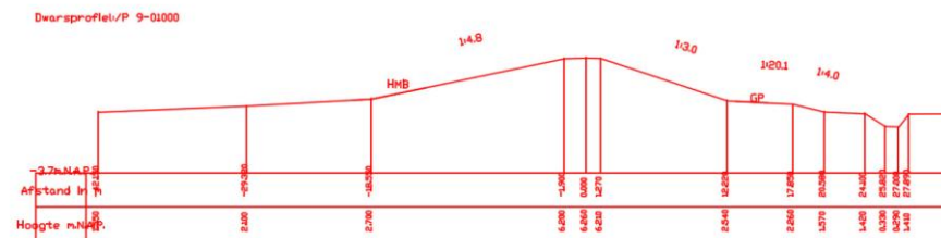
Figuur 7 Huidig dwarsprofiel ter hoogte van km 13
