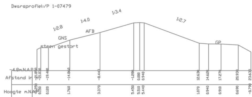
Figuur 12 Actuele hoogte, NAP + 5.5 m, hoogte 1943, NAP + 5.11 (km #4.5)
