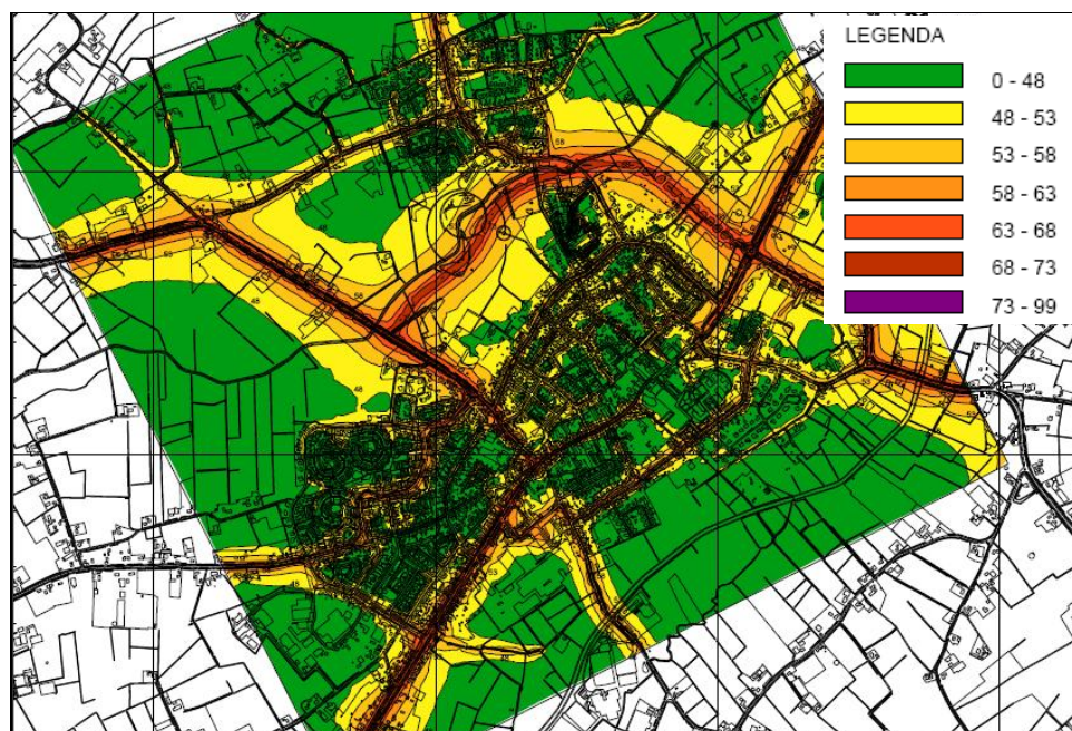
Figuur 6.17 Geluidbelasting wegverkeer alternatief 1a (dB)
