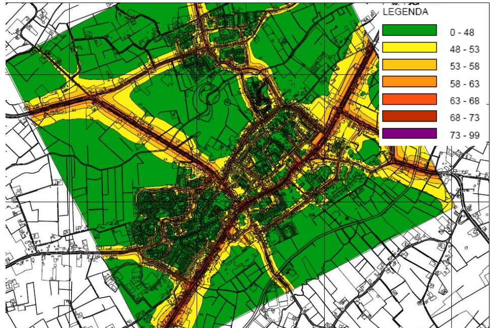
Figuur 4.23 Geluidbelasting wegverkeer huidige situatie (dB)
