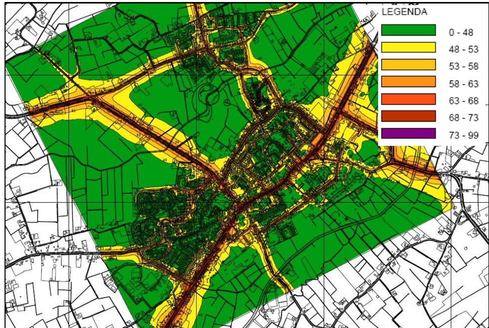
Figuur 2.1 Geluidbelasting wegverkeer huidige situatie (dB)
