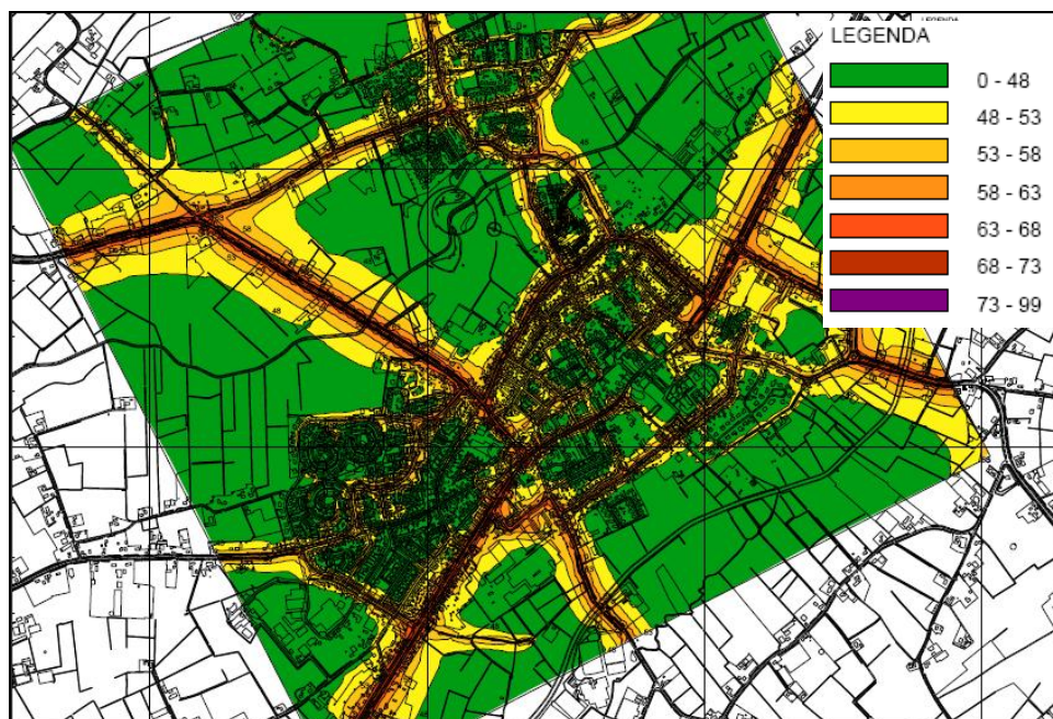
Figuur 4.24 Geluidbelasting wegverkeer autonome situatie (dB)
