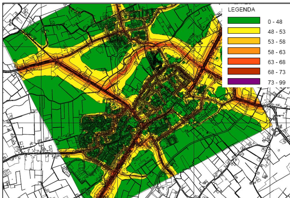
Figuur 6.19 Geluidbelasting wegverkeer alternatief 1b (dB)
