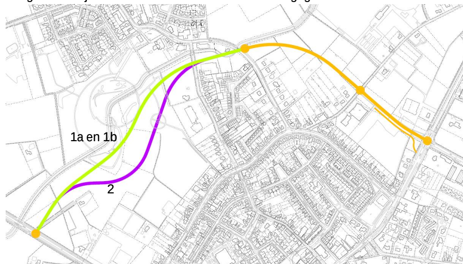
Figuur 5.6 De tracés voor de Randweg
