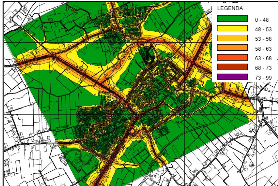
Figuur 6.21 Geluidbelasting wegverkeer alternatief 2 (dB)
