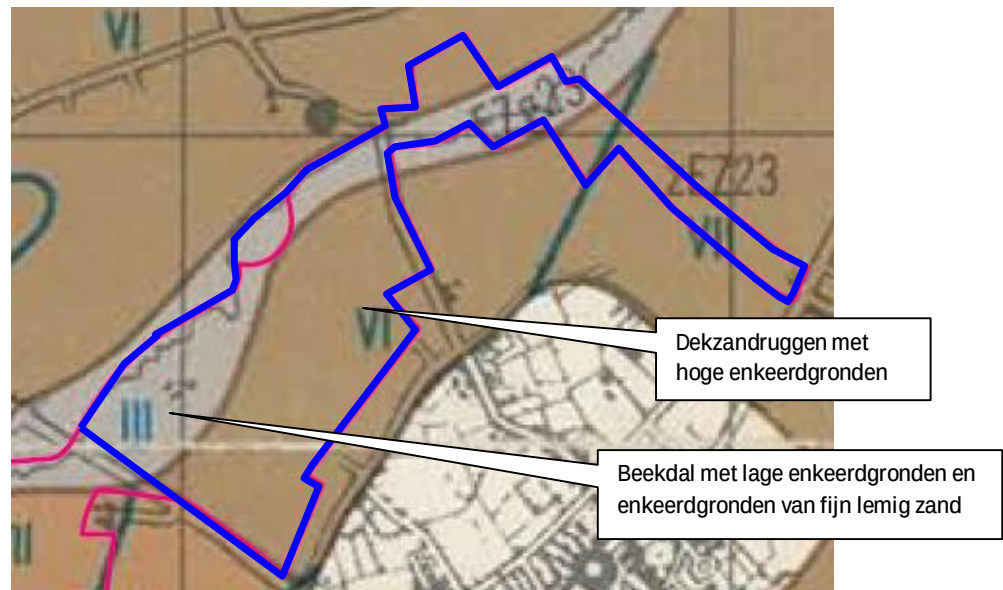
Figuur 4.7 Bodemtype (bron: Stiboka/Compositie 5, 2007)
