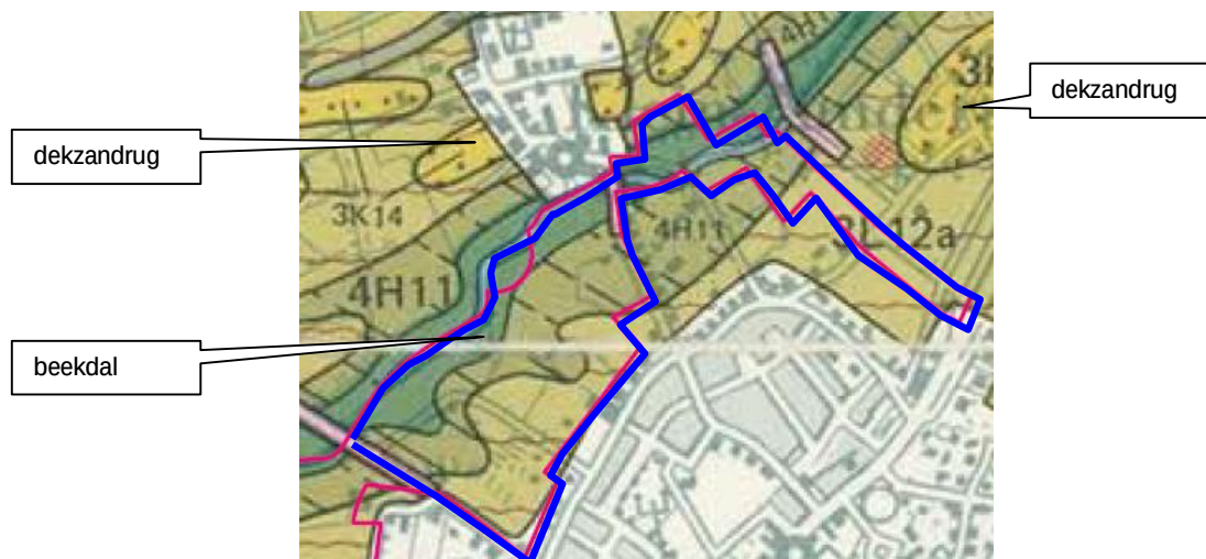
Figuur 4.4 Landschappelijke opbouw / geomorfologie (bron: Compositie 5, 2007)
