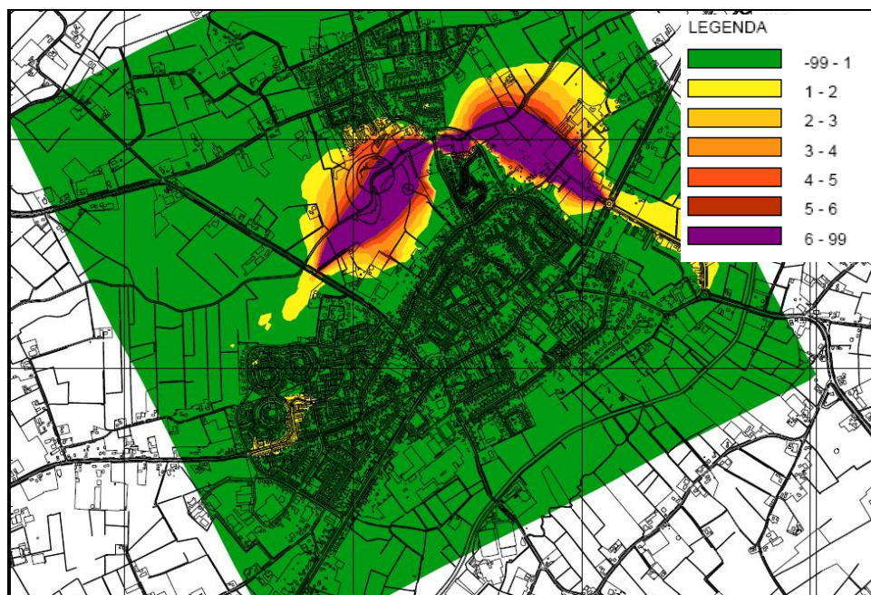
Figuur 6.20 Verschil geluidbelasting wegverkeer alternatief 1b versus autonome situatie (dB)
