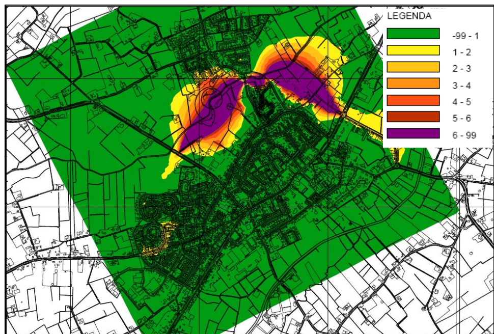
Figuur 6.22 Verschil geluidbelasting wegverkeer alternatief 2 versus autonome situatie (dB)
