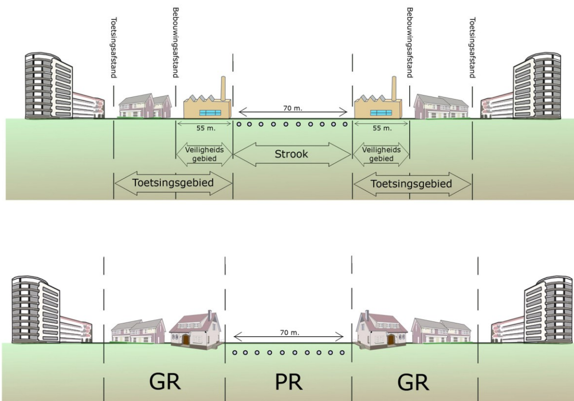
Figuur 8.4. Figuur met veiligheidsafstanden Structuurvisie buisleidingen
