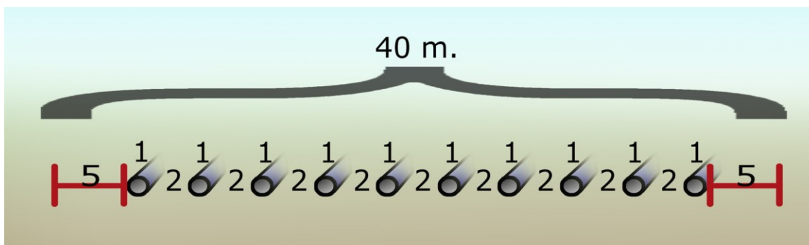
Figuur 8.2. Dwarsdoorsnede leidingenstrook van 40 meter met buisleidingen op onderlinge afstand van 2 meter
