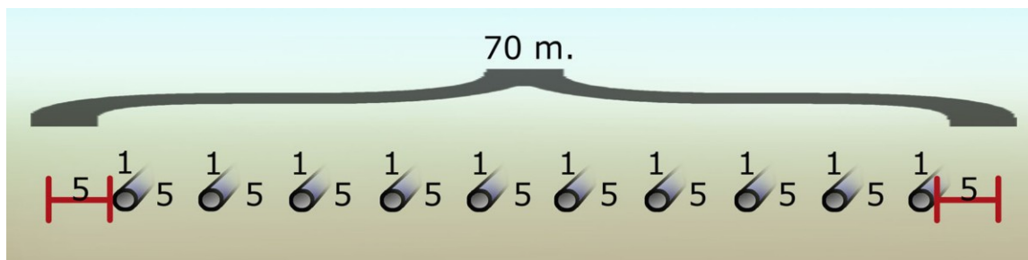
Figuur 8.1. Dwarsdoorsnede leidingstrook van 70 meter met buisleidingen op onderlinge afstand van 5 meter
