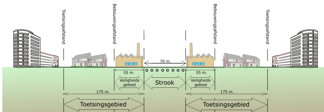
Figuur 2.5. Overzicht met veiligheids- en toetsingsgebieden SBUI
