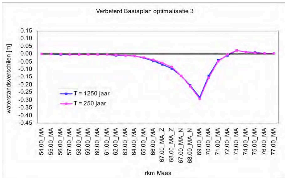
Waterstandsverandering 1/1.250 jaar afvoer en 1/250 jaar afvoer bij het Verbeterd Basisplan (inclusief optimalisatie 3) ten opzichte van de actuele situatie (Wijbenga & Vieira da Silva, 2010).
