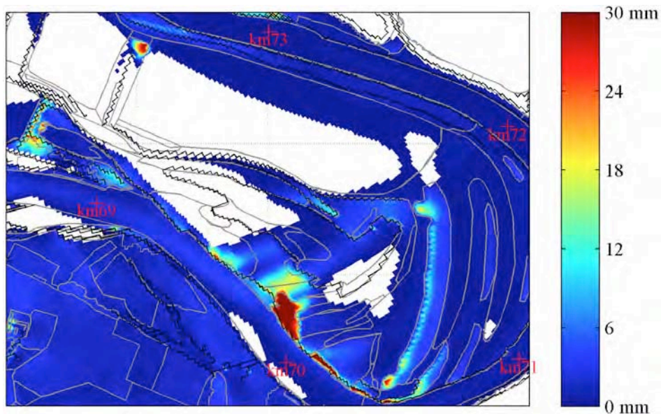
Korrelgrootte die in beweging komt bij de 1/250 jaar afvoer, Variant Ganzengrasland (Wijbenga & Vieira da Silva, 2010).
