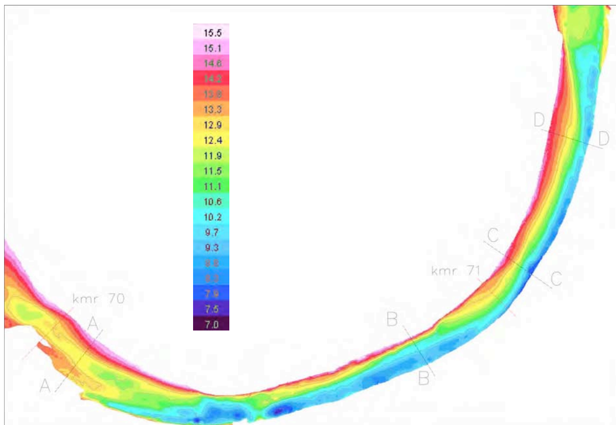
Huidige bodemligging van de Maas. Peiling zomer 2009 in meters +NAP. Stuwpeil is 16,90 m+NAP. (Dibec, 2009).
