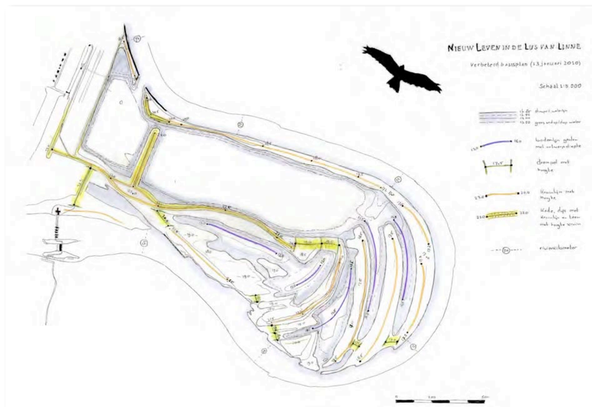
Verbeterd Basisplan. Contouren en ontwerphoogtes (eindbeeld).
