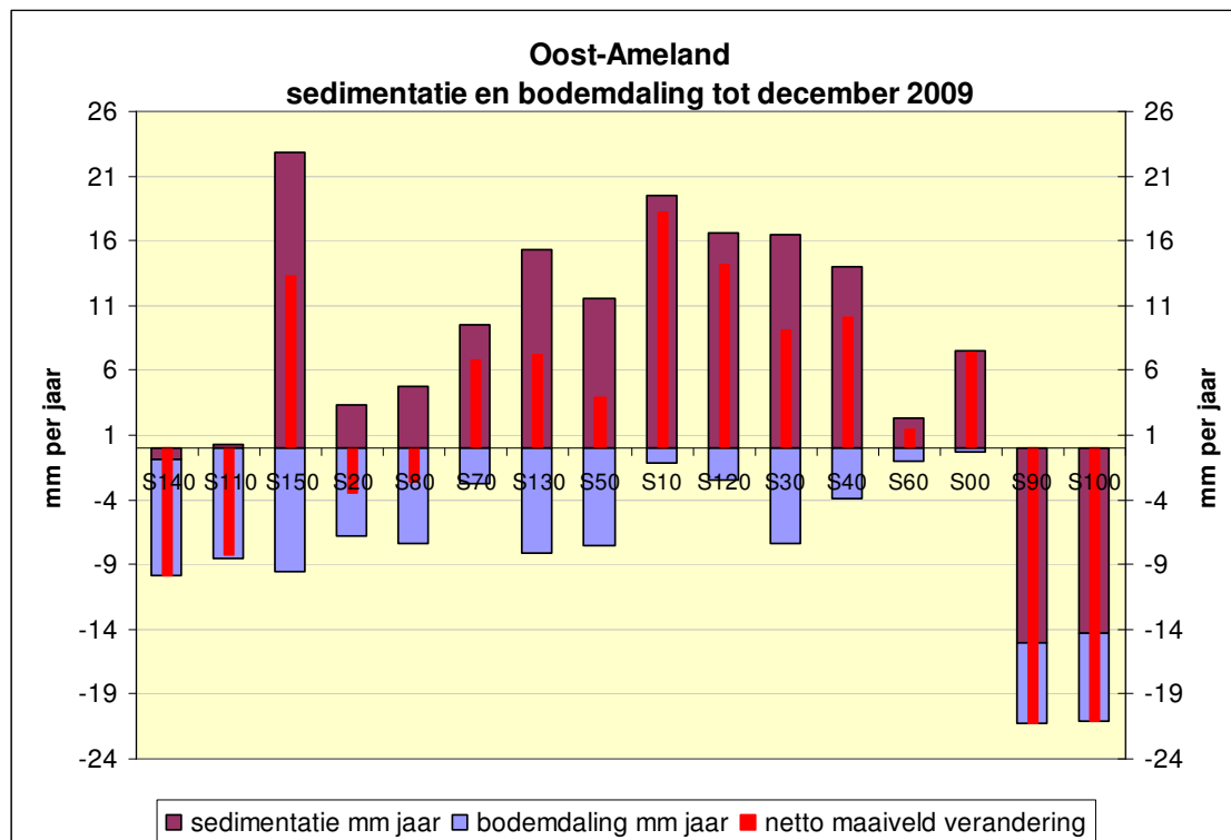
Figuur 22. Netto gemiddelde sedimentatie/erosie per jaar gedurende de gehele meetperiode per meetstation. Bijgewerkt tm december 2009. De bodemdaling is niet exact en definitief. Hiervoor vindt nog een herberekening plaats in de loop van 2010.
