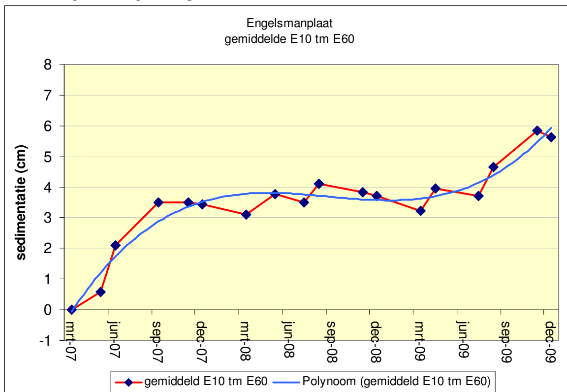
Figuur 13. Gemiddelde van de gemiddeldes van meetstations E10 tm E60 in het onderzoeksgebied Engelsmanplaat.
