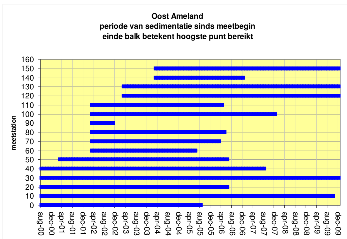
Figuur 23. Oost-Ameland. Grafische weergave van periode van begin van meting tot de hoogst gemeten waarde. Daarna volgt tenminste erosie tot eind van de meetreeks in december 2009.
