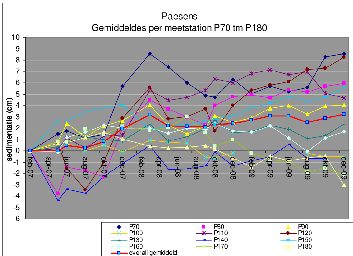
Figuur 10. Gemiddelde meetlijnen van de meetstations P70 tm P180 in het onderzoeksgebied bij Paesens. Tevens is het gemiddelde van deze 12 meetlijnen genomen als weergave van de sedimentatie van het gebied waarin de meetstations liggen.
