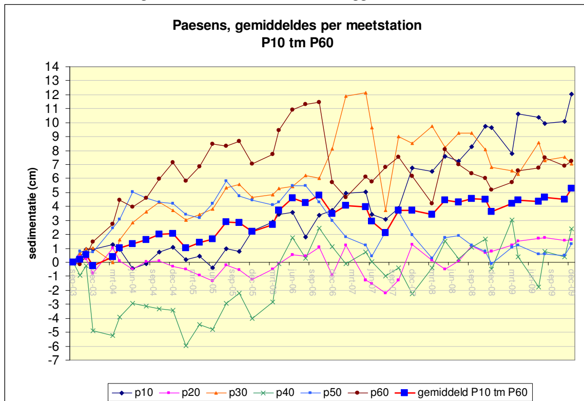
Figuur 9. Gemiddelde meetlijnen van de meetstations P10 tm P60 in het onderzoeksgebied bij Paesens. Tevens is het gemiddelde van deze 6 meetlijnen genomen als weergave van de sedimentatie van het gebied waarin de meetstations liggen.
