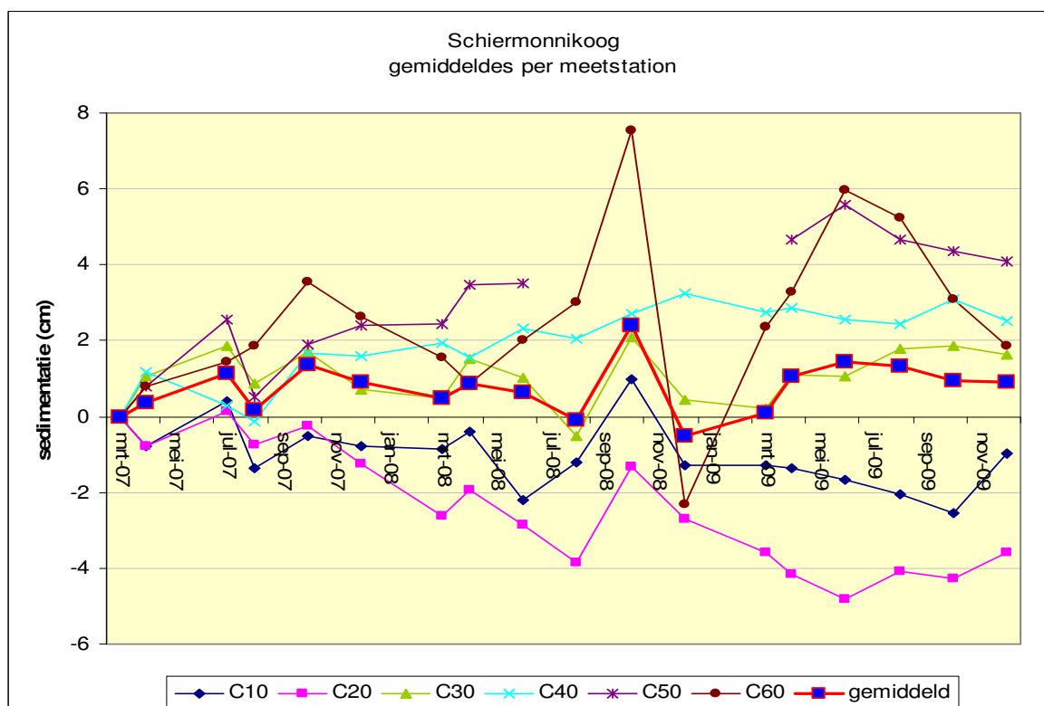
Figuur 14. Gemiddelde meetlijnen van de meetstations C10 tm C60 in het onderzoeksgebied Schiermonnikoog. Tevens is het gemiddelde van deze 6 meetlijnen genomen als weergave van de sedimentatie van het gebied waarin de meetstations liggen.
