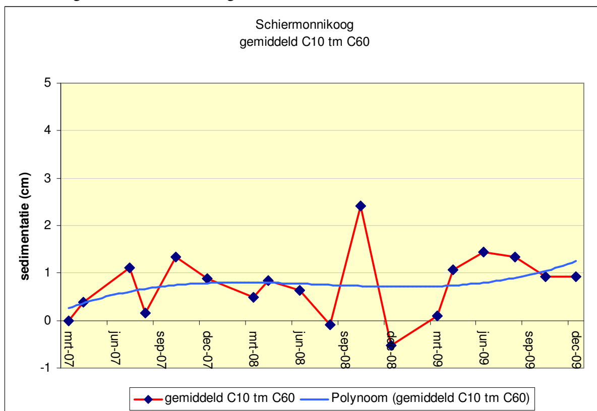
Figuur 15. Gemiddelde van de gemiddeldes van de meetstations C10 tm C60 in het onderzoeksgebied Schiermonnikoog.
