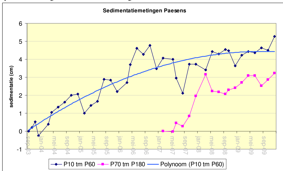
Figuur 11. Gemiddelde van de gemiddeldes van meetstations P10 tm P60 en P70 tm P180 in het onderzoeksgebied bij Paesens. De lijn P70 tm P180 is herberekend en gecorrigeerd ten opzichte van de grafiek in het 2008 verslag.
