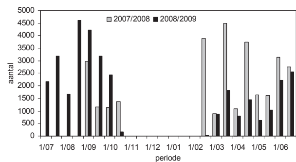
Figuur 6. Aantallen steltlopers en sterns op slaappleatsen in het Lauwersmeergebied in de periode begin juli 2008-eind juni 2009, (waarbij 1/9 = 1 e helft september; 2/9 = 2 e helft september; enz.), in vergelijking met het seizoen 2007/2008. In het seizoen 2007/2008 zijn in de periode 1/07-2/08 (juli-augustus) geen tellingen uitgevoerd. Vanaf het seizoen 2008/2009 worden geen tellingen meer uitgevoerd in de periode 1/11-1/02 (begin november-begin februari).
