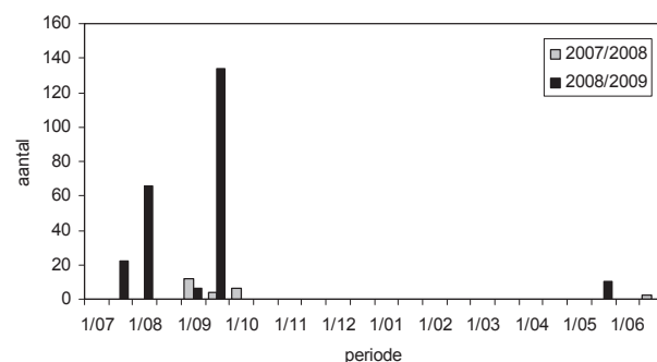
Figuur 44. Seizoenspatroon van de Kleine Strandloper op slaapplekken in het Lauwersmeergebied in de seizoenen 2007/2008 en 2008/2009, in de periode juli-juni. In het seizoen 2007/2008 zijn geen tellingen uitgevoerd in juli en augustus (1/07-2/08). In de periode november-eerste helft februari zijn geen slaapplekstellingen uitgevoerd (1/11-1/02).
