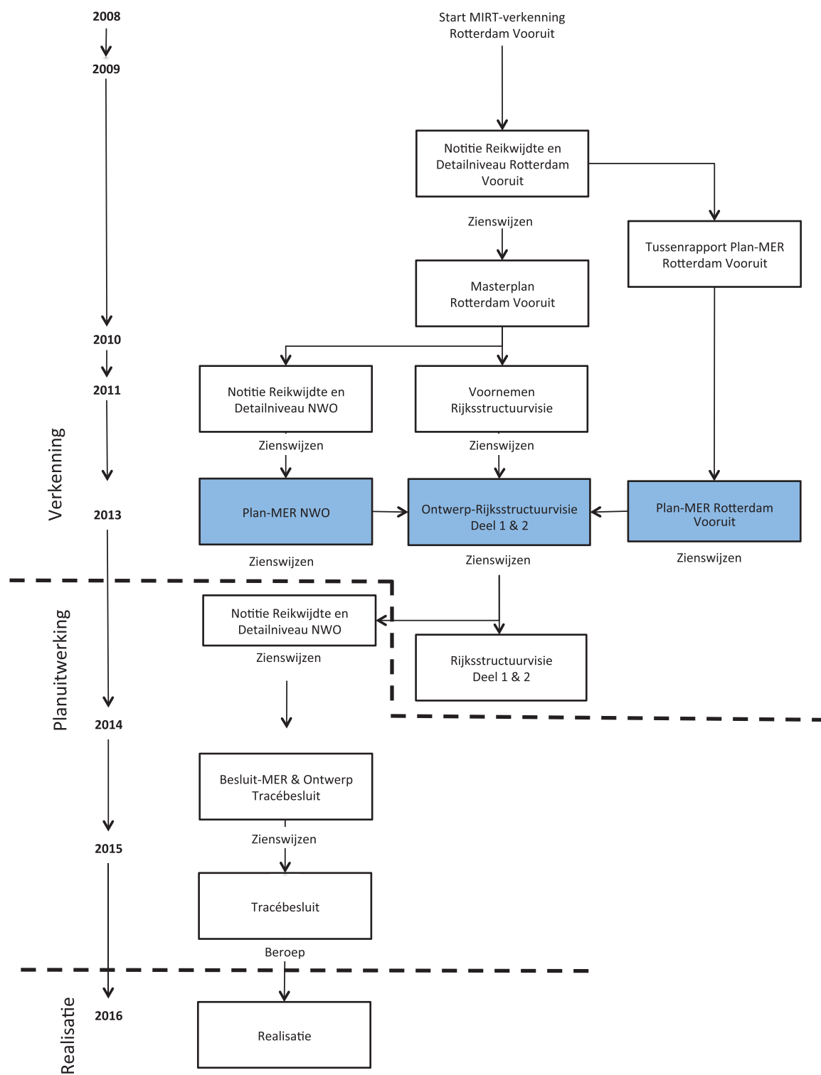
Figuur 2. Procedureschema
