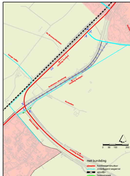
Figuur 4.3: Bundelen tracé Traverse met spoorlijn
