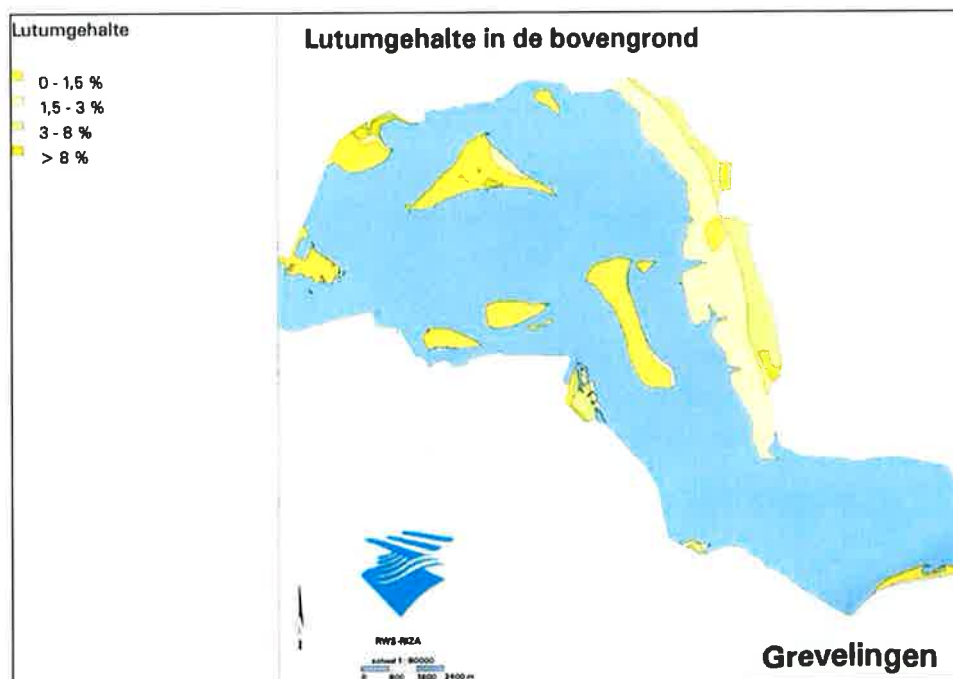
Figuur 4. Lutumgehaltes in de bovengrond (Bron: RWS, RIZA). Lutum zijn de gronddeeltjes kleiner dan 2 \mu\text{m} . Bodems met minder dan 5% lutum worden klei-arm zand genoemd, tussen 5 en 8% kleilig zand, boven 8% lutum is sprake van zavel en boven 25% spreekt men van klei (Stiboka 1987).
