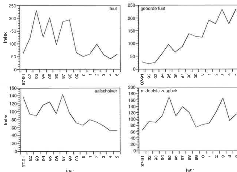
Afbeelding 3. Indices van vier viseters in de Grevelingen in de periode 1987-2005. Het gemiddelde aantal vogeldagen over de gehele periode is op 100 gesteld. Voor de seizoenen 1987-1991 is de gemiddelde index gegeven. Bron: Strucker et al. (2007).
