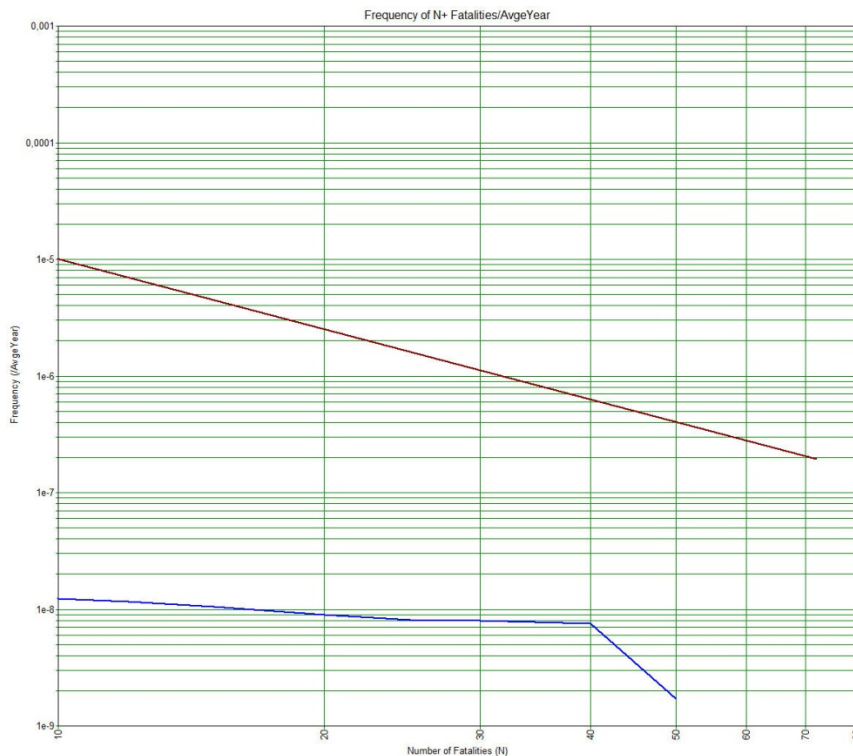
Figuur 5.2 Groepsrisico RWZI 's-Hertogenbosch
