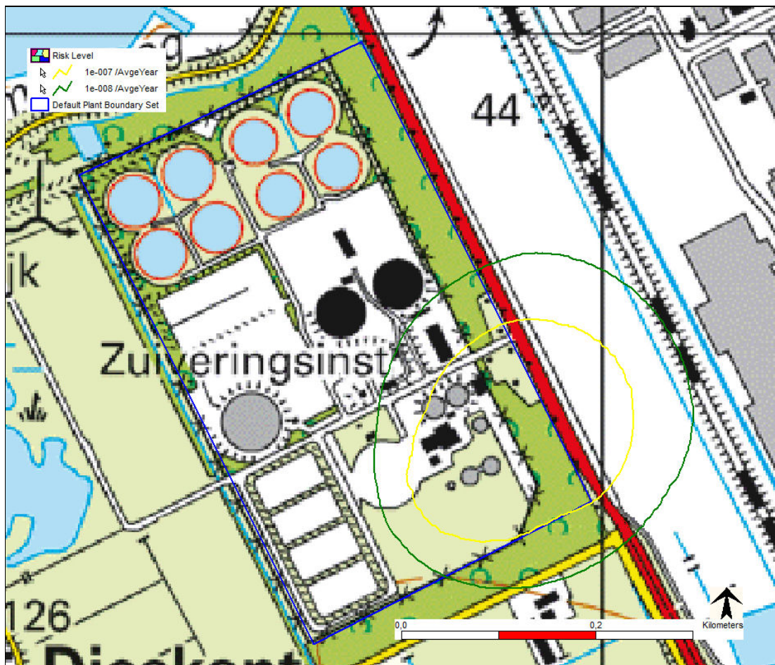
Figuur 5.1 Plaatsgebonden risico RWZI 's-Hertogenbosch
