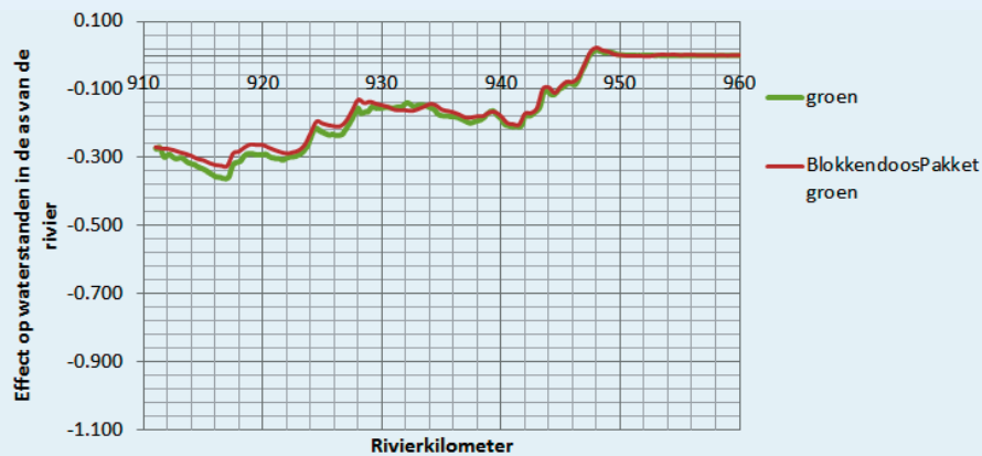
Afbeelding 10: Vergelijking waterstandseffect van de alternatieven berekend met de Blokkendoos en met een Pakketsom (linksboven = alternatief blauw, rechtsboven = alternatief blauw light, linksonder = alternatief groen, rechtsonder = alternatief rood)
