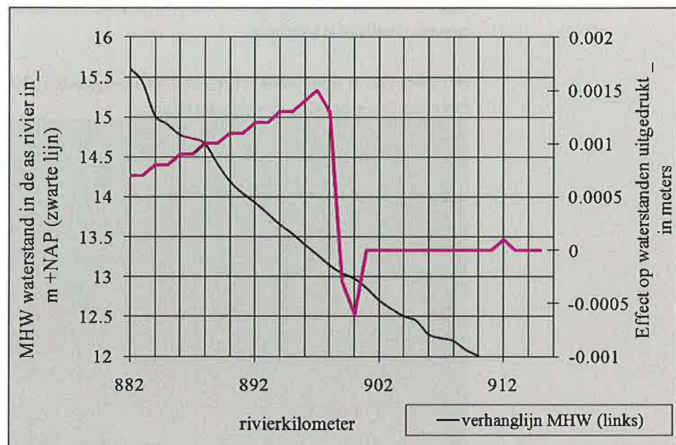
Figuur 2. De zwarte lijn met de bijbehorende linker y as geeft de waterhoogte weer, de paarse lijn met de bijbehorende rechter y as geeft het effect van de ingreep weer. De verhoogde toegangsweg geeft tot 1,5 mm opstuwing in de rivier. Referentie: Simona_rijn_pkb_3_2 opgenomen in maptable 2.0.
