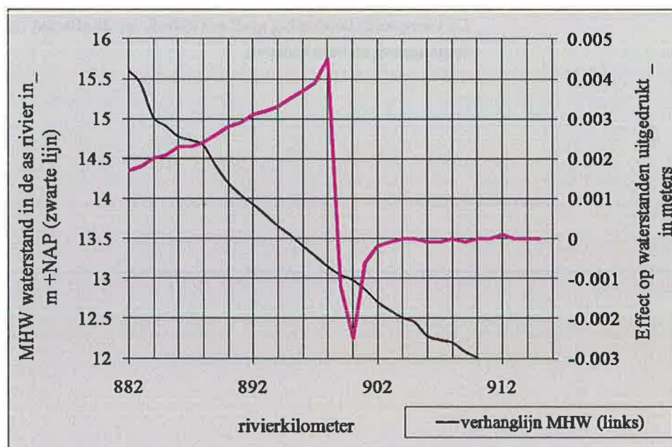
Figuur 7. De zwarte lijn met de bijbehorende linker y as geeft de waterhoogte weer, de paarse lijn met de bijbehorende rechter y as geeft het effect van de ingreep weer. Het maximale effect van Alternatief A bedraagt hier 4,5 mm. Referentie: Simona_rijn_pkb_3_2 opgenomen in maptable 2.0.
