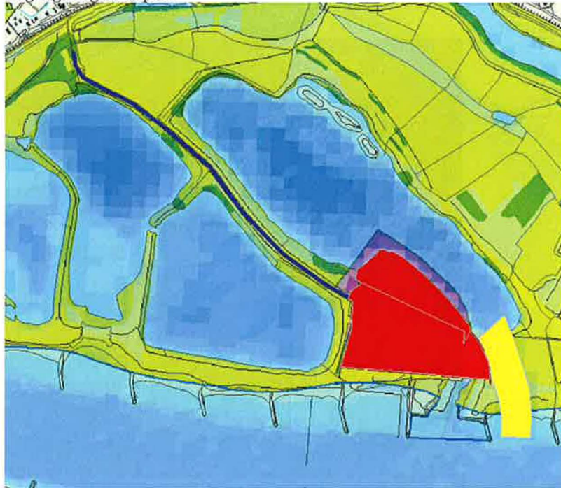
Figuur 15. In rood, geel en blauw de ingetekende ophoging alternatief B, met invaartopening, toegangsweg en depot. Paars is ophoging alternatief A, groen is ondergrond.
