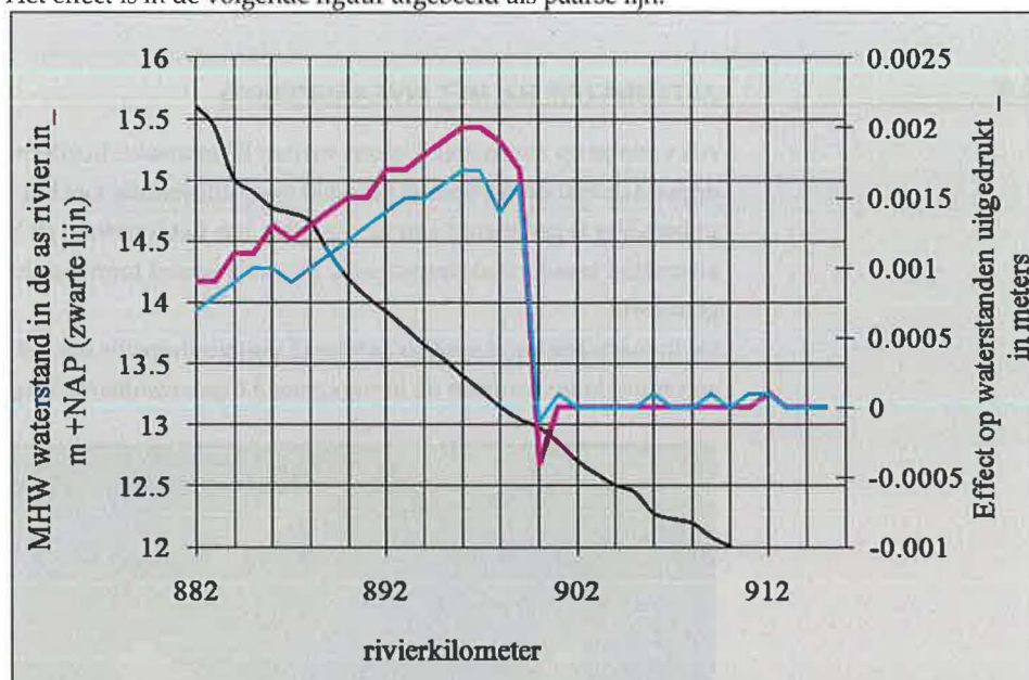
Figuur 19. De zwarte lijn met de bijbehorende linker y as geeft de waterhoogte weer, de paarse lijn met de bijbehorende rechter y as geeft het effect van de ingreep weer. Het maximale effect van alternatief B2 bedraagt 2 mm met kleidepot. Hierbij is nog geen rekening gehouden met het feit dat het kleidepot ook in de huidige situatie aanwezig is. Referentie: Simona_rijn_pkb_3_2 opgenomen in maptable 2.0. Als daarmee wel rekening wordt gehouden is het effect 1.5 mm dit is afgebeeld als een blauwe lijn.
