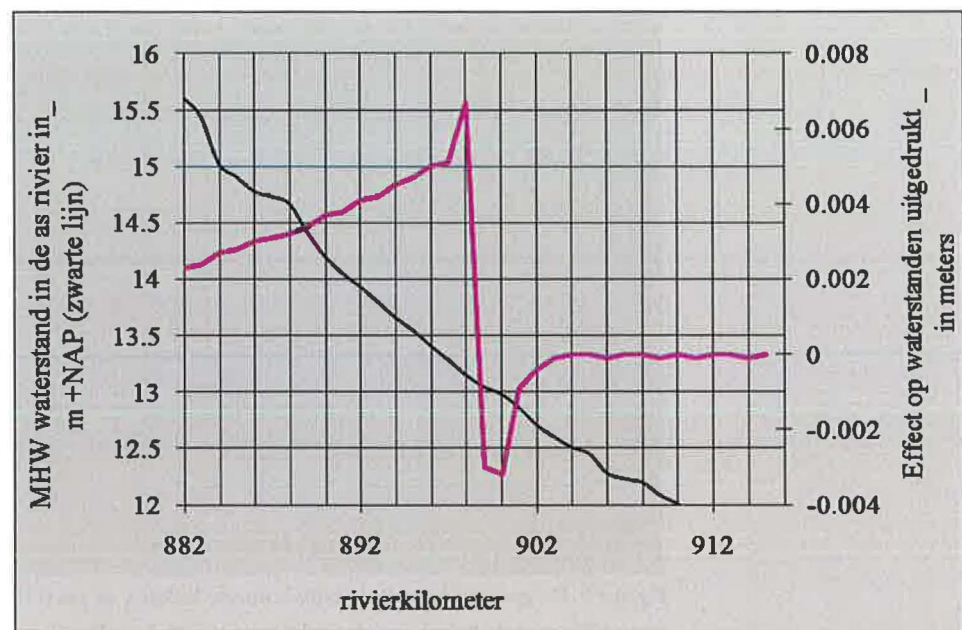
Figuur 11. De zwarte lijn met de bijbehorende linker y as geeft de waterhoogte weer, de paarse lijn met de bijbehorende rechter y as geeft het effect van de ingreep weer. Het maximale effect van Alternatief B zonder inlaat bedraagt hier ca 6,5 mm. Referentie: Simona_rijn_pkb_3_2 opgenomen in mactable 2.0.
