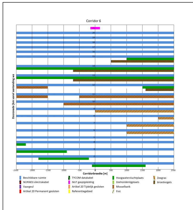
Figuur 9 Bovenaanzicht per kilometer van corridor 6
