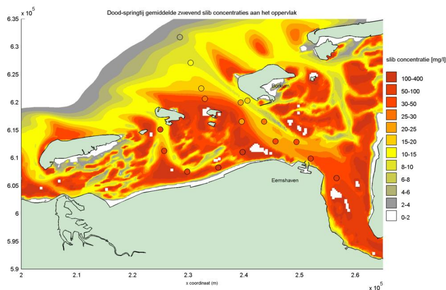
Figuur 34 Ruimtelijke verdeling van de zwevend slib concentraties gemiddeld over een doortij-springtij cyclus [MER Windparken GEMINI, 2012].
