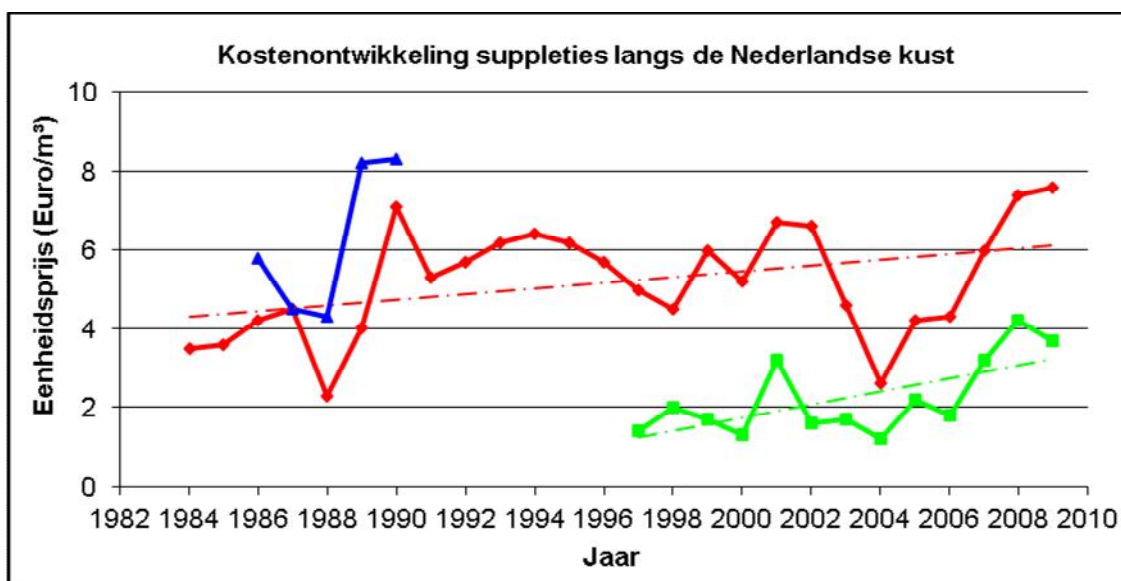
Figuur 24 Gemiddelde eenheidsprijs voor zandsuppleties langs de Nederlandse kust per m³ in de afgelopen 30 jaar
