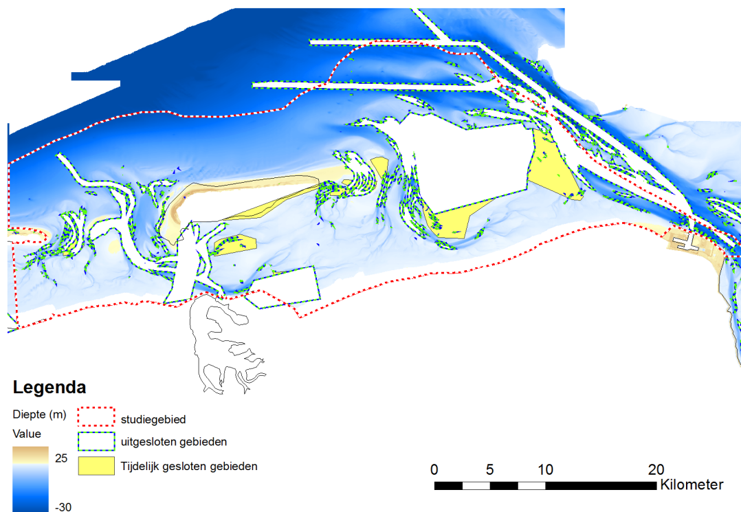
Figuur 3 Alle verzamelde uitgesloten en problematische gebieden binnen het studiegebied.
