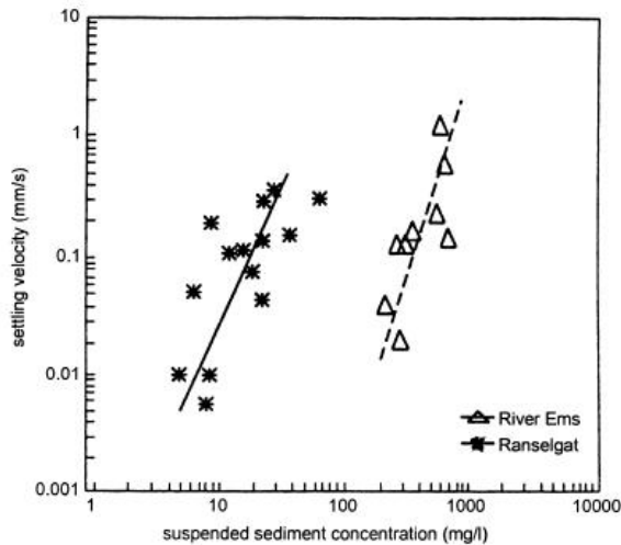
Figuur 32 Valsnelheid als functie van sediment concentratie (Van Leussen, 1999)
