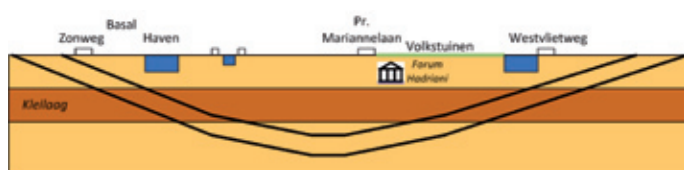
figuur 5.1 Schematisch overzicht van de verticale ligging van de Boortunnel
