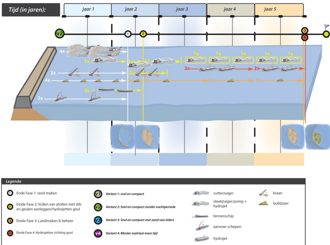
Figuur 5.7: Inzet materieel voor de eerste fase van 500 hectare bij de variant 'snel en compact zonder nacht'
