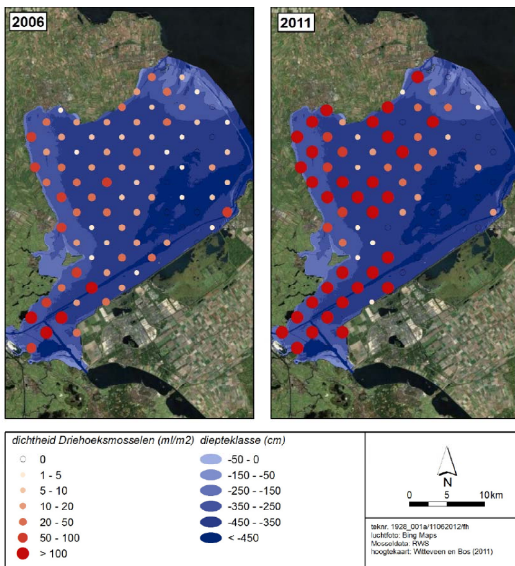
Figuur 3.18: Driehoeksmosselen in het Markermeer en IJmeer in 2006 en 2011. Figuur afkomstig uit Witteveen en Bos, 2012
