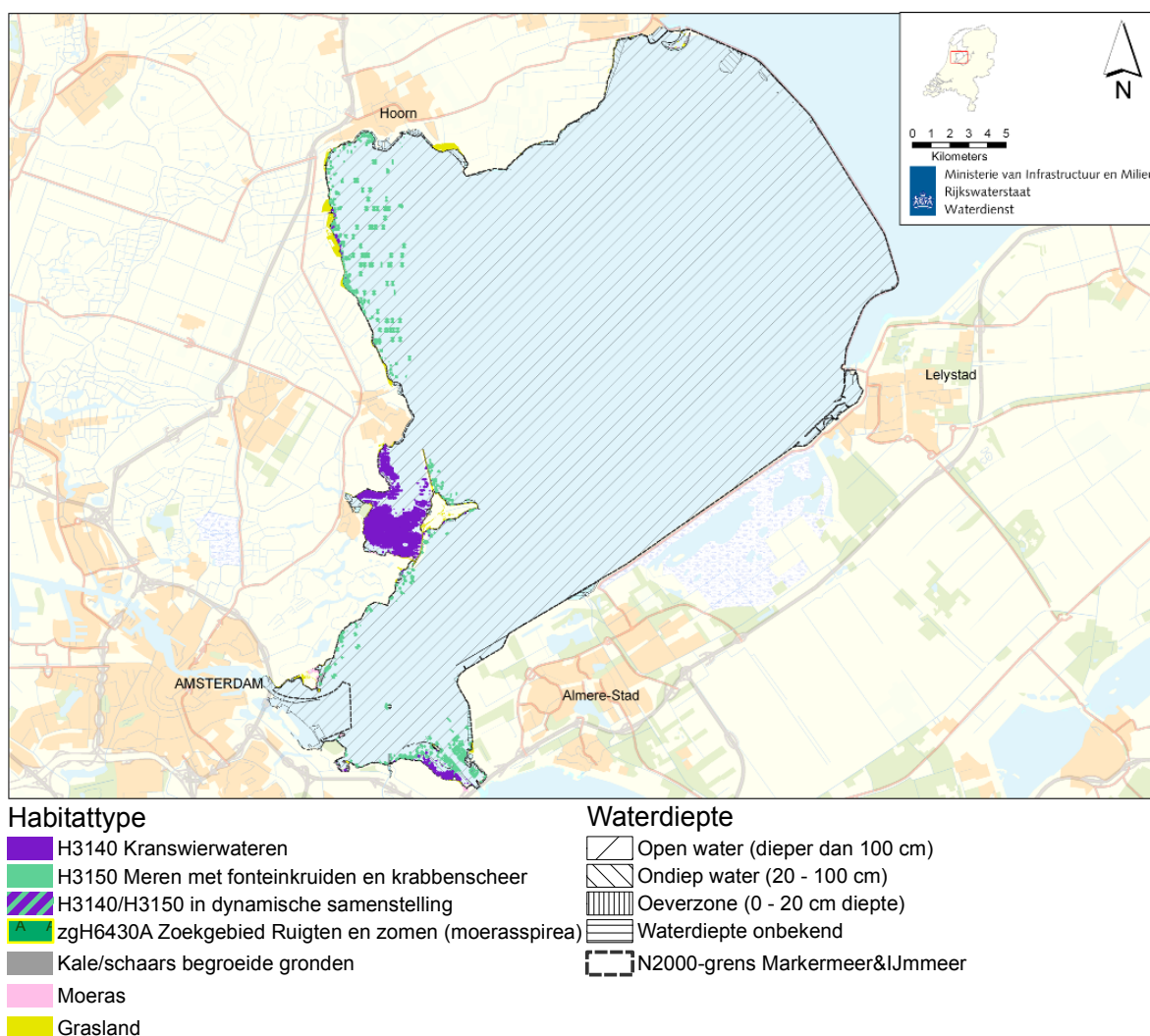
Figuur 3.3: Verspreiding van habitattypen in het Markermeer. ( www.natura2000ijsselmeergebied.nl )
