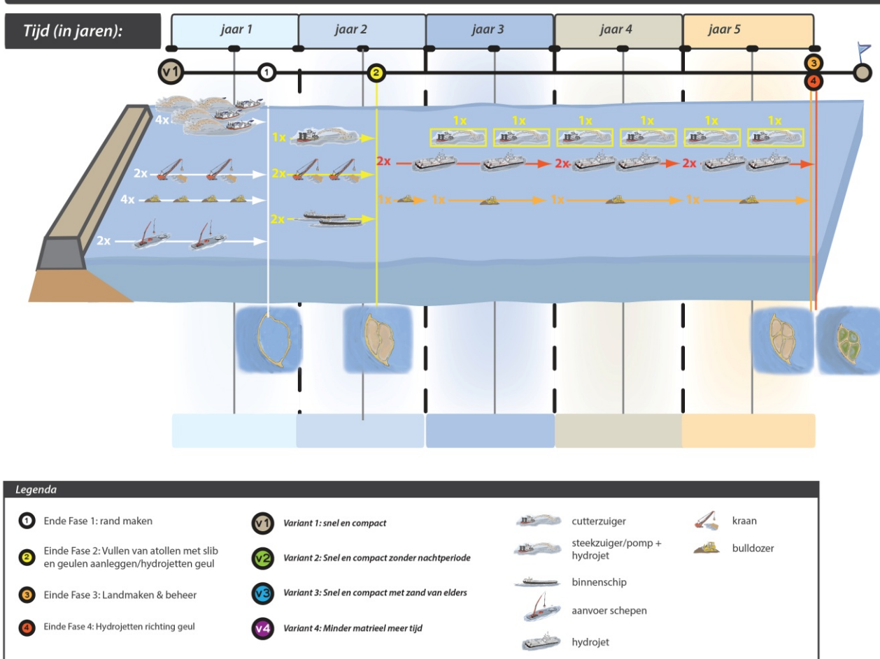
Figuur 5.6: Inzet materieel voor de eerste fase van 500 hectare bij de variant 'snel en compact'
