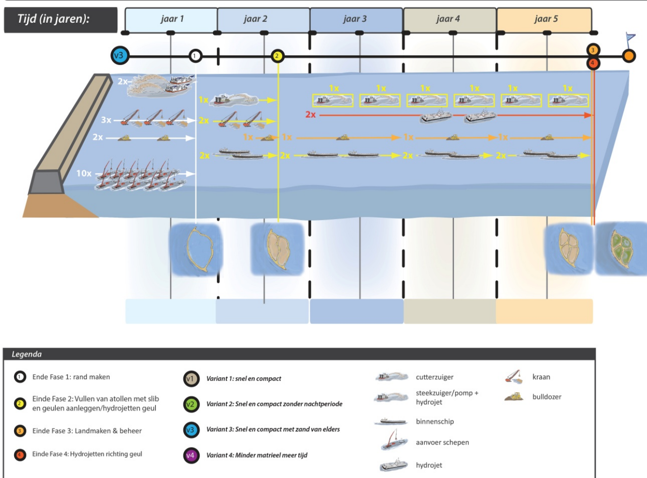
Figuur 5.8: Inzet materieel voor de fase van 500 hectare bij de variant 'snel en compact met zand van elders'
