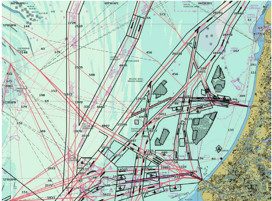
Figuur 5-6 Verkeersafwikkeling (niveau 2008) bij het windgebied HK voordat er windturbines geplaatst zullen worden
