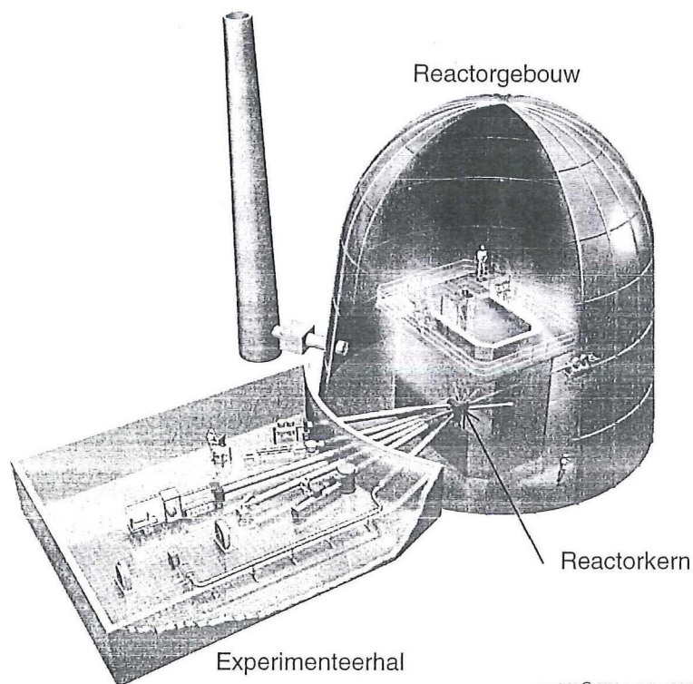
Figuur 1 Doorsnede van het reactorgebouw en de experimenteerhal
