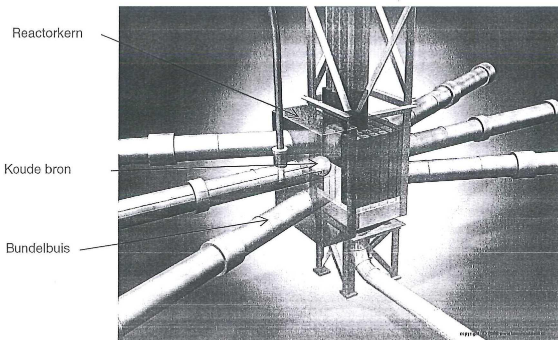
Figuur 2 Reactorkern met bundelbuizen en koude bron
