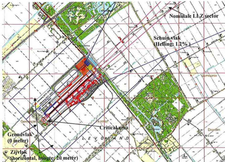
Figuur 3.1 Critical area, toetsvlakken, nominale LLZ sector en obstakels in geval van een Localizer installatie voor een straight-in nadering.
