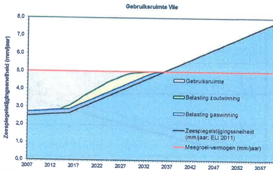
Figuur 1: Gebruiksruimte kombergingsgebied Vlie, uitgaande van een meegroeivermogen van 5 mm/jaar en het nieuwe TNO-scenario voor zeespiegelstijging. Over de gehele lengte van de gebruiksruimte is rekening gehouden met een belasting van 0,22 mm/jaar vanwege de bestaande gaswinning Zuidwal (0,12 mm/jaar) en mogelijk toekomstig Pollendam (0,10 mm/jaar). De verwachte belasting van de gebruiksruimte door de toekomstige zoutwinning van Frisia is door de groene lijn aangegeven (periode 2015-2034). Hierbij over 6 jaarlijks gemiddeld volgens protocol.
