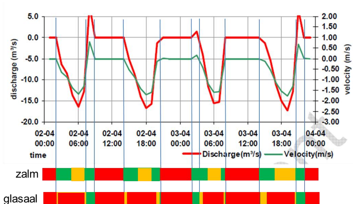
Figuur 4-5: In de VMR haalbaarheidsstudie heeft Deltares stromingsomstandigheden in de koker gemodelleerd. Op basis hiervan zijn de migratievensters van zalm (sterke zwemmer) en glasaal (zwakke zwemmer die vooral selectief getijdetransport zal benutten) weergegeven. Rood geeft aan dat migratie niet mogelijk is; aanvullende stroming remmende voorzieningen zijn dan nodig. Groen geeft aan dat migratie zeker mogelijk is. Oranje geeft aan dat migratie wellicht mogelijk is (voor zalm is dit afhankelijk van de lengte van de zalm en de watertemperatuur; voor glasaal of deze naast selectief met de stroming mee ook via actief zwemmen de koker kan passeren).
