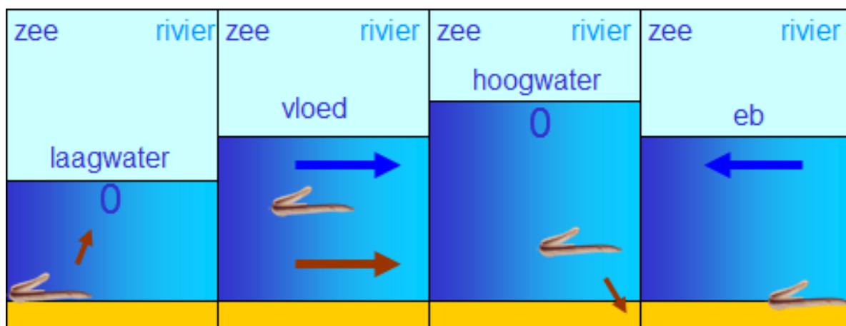
Figuur 4-2. Een grafische voorstelling van selectief getijdetransport. Tijdens afgaand tijd drukt vis zich tegen de bodem om positie te houden en tijdens opkomend tij wordt de waterkolom opgezocht om energetisch efficiënt gebruik te maken van de waterstroom
