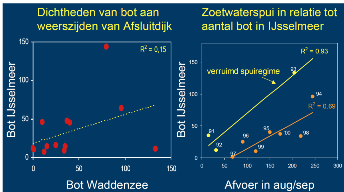
Figuur 4-6. Dichtheden bot in het IJsselmeer in relatie tot dichtheden op de Waddenzee over de periode 1991-2000 (linker paneel) en de hoeveelheid gespuide water, waarbij onderscheid is gemaakt tussen jaren met het 'normale' spuiregime en de jaren 1991-93 (weliswaar n=3 , maar allen boven de andere waarden) waarin er per getij iets langer is gespuide (tot gelijk waterniveau i.p.v. 10 cm beneden IJsselmeerpeil). Uit Winter (2009).
