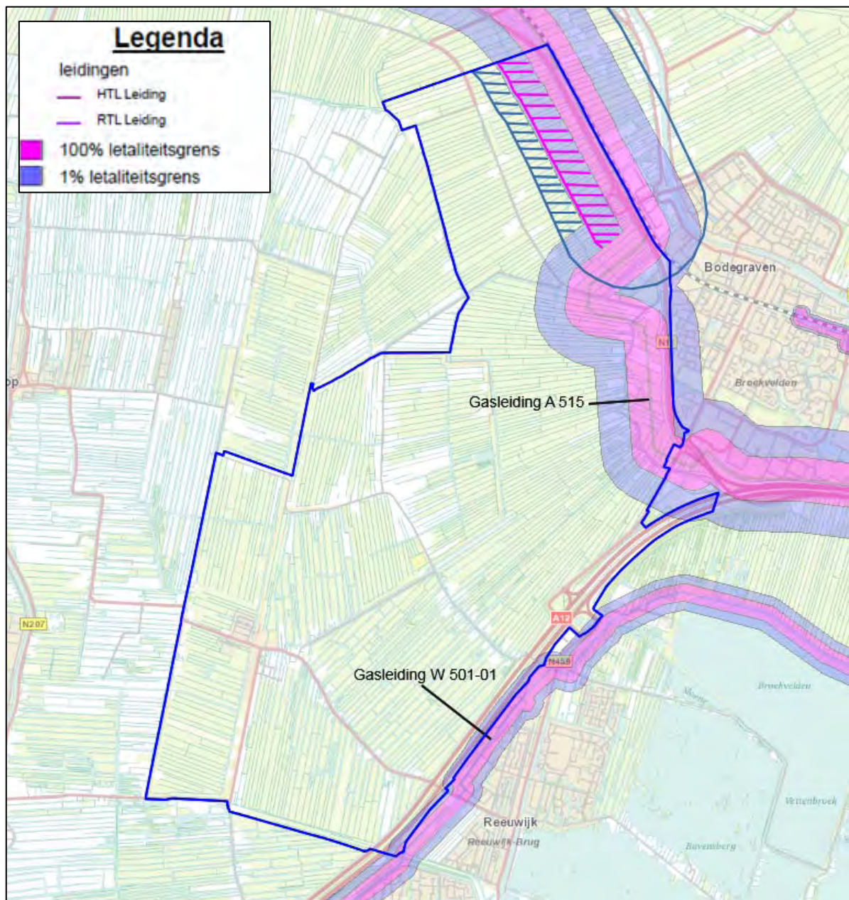
Figuur 5: Gasleidingen met invloedsgebieden en 100% letaalzone
