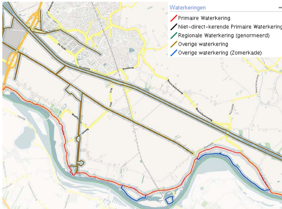
Figuur 7.5 Waterkeringen
