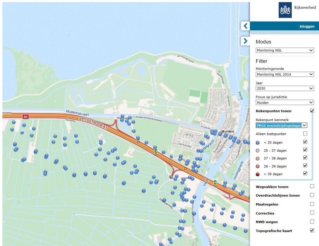
Figuur 68: PM 10 overschrijdingsdagen Muiden in 2030
