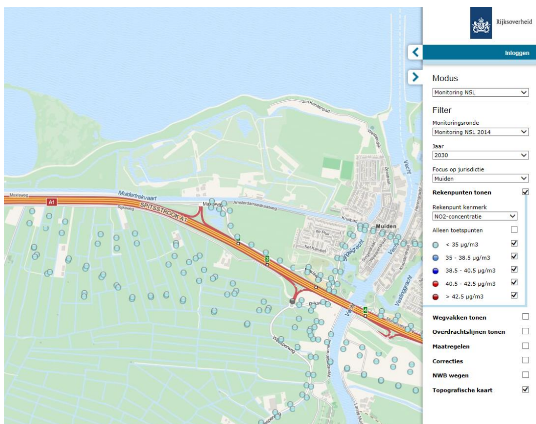
Figuur 67: NO 2 concentratie Muiden in 2030
