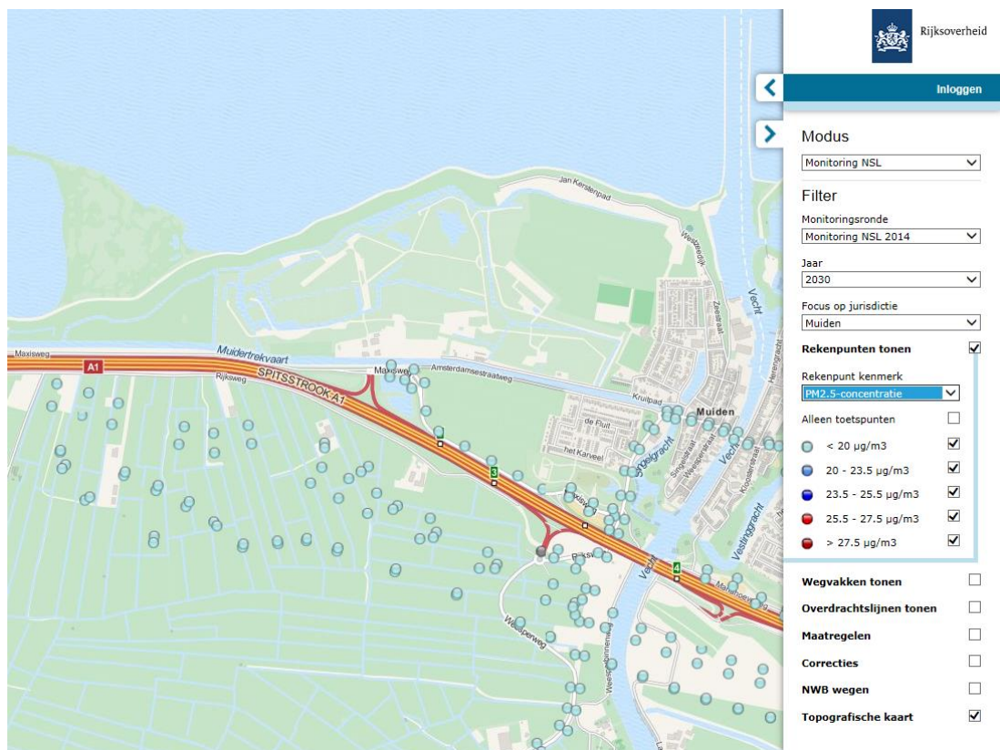
Figuur 69: PM 2,5 concentratie Muiden in 2030
