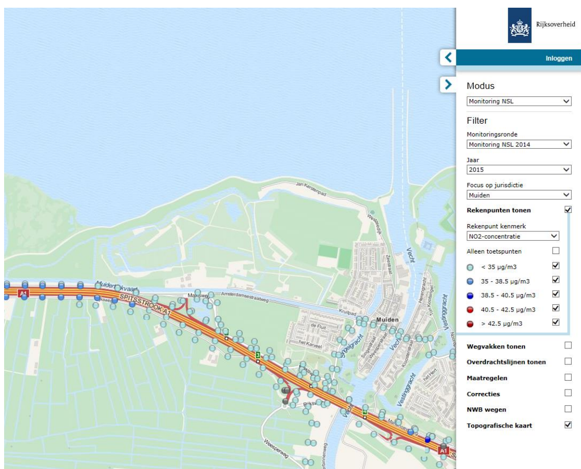
Figuur 64: NO 2 concentratie Muiden (RWS, 2015)
