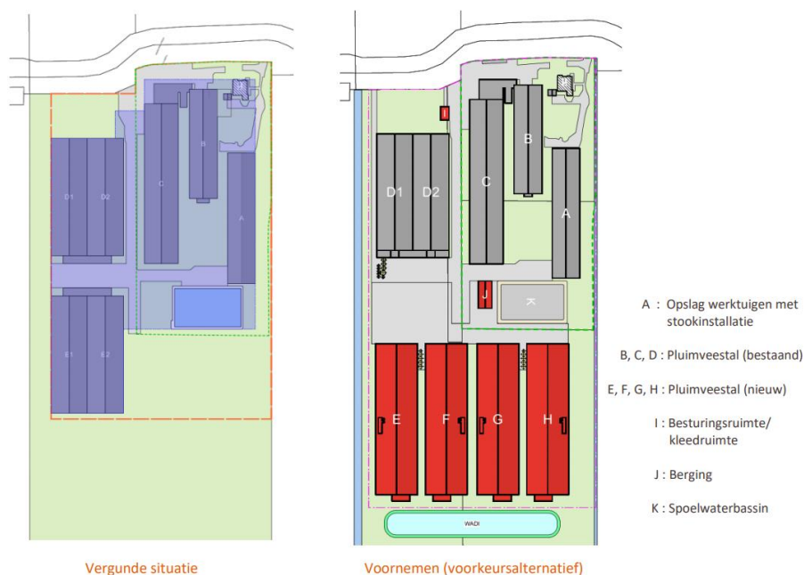
Afbeelding 1 Vergunde situatie (zoals voor de brand gerealiseerd was) en de beoogde situatie (bron: Aanvulling).
