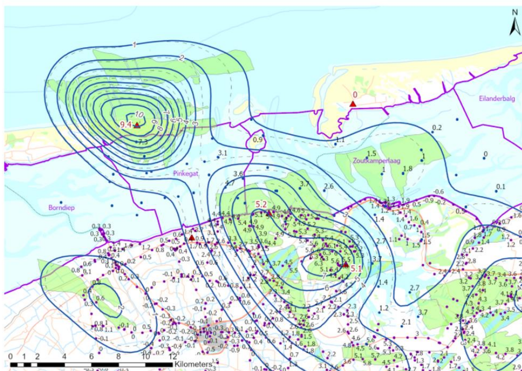
Figuur 3: Schatting van de diepe-bodemdaling door gaswinning in het Waddengebied sinds de nulmeting in 2006 (in centimeters) tot eind 2021. Gaswinning vindt sinds 1986 plaats bij Ameland en sinds 2007 in de gaswinningsgebieden Moddergat, Lauwersoog en Vierhuizen. In blauw de contouren van de gemodelleerde diepe-bodemdaling volgens het verwachte scenario. De gestreepte contouren geven de diepe-bodemdaling van 2020 weer uit de rapportage over de Meet & Regelcyclus 2020. De blauwe punten met label in de Waddenzee representeren de peilmerken met de gemeten hoogteverschillen vanaf 2006 tot de meting in mei 2021, en de paarse punten met label op het vaste land representeren de peilmerken met de met InSAR gemeten hoogteverschillen vanaf eind 2006 tot eind 2020. De rode waarden geven de daling aan van de permanente GPS-stations in de periode februari 2007–december 2021. Bron: NAM-rapport EP202204201384 – figuur 6.
